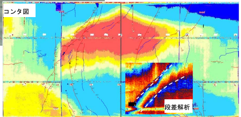
図-4 覆工内面への変形箇所
