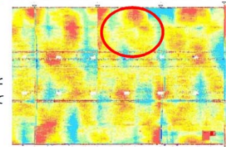
当初ひび割れ展開図より 縦断方向に1.0mm程度のひび割れがあり、斜め方向のひび割れとつながると将来閉合する恐れがあるものと判断していた
