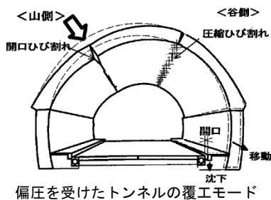
図-4 覆工内面への変形箇所
