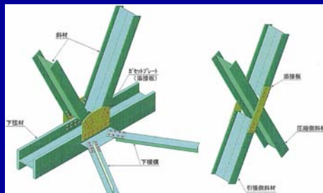
格点構造
