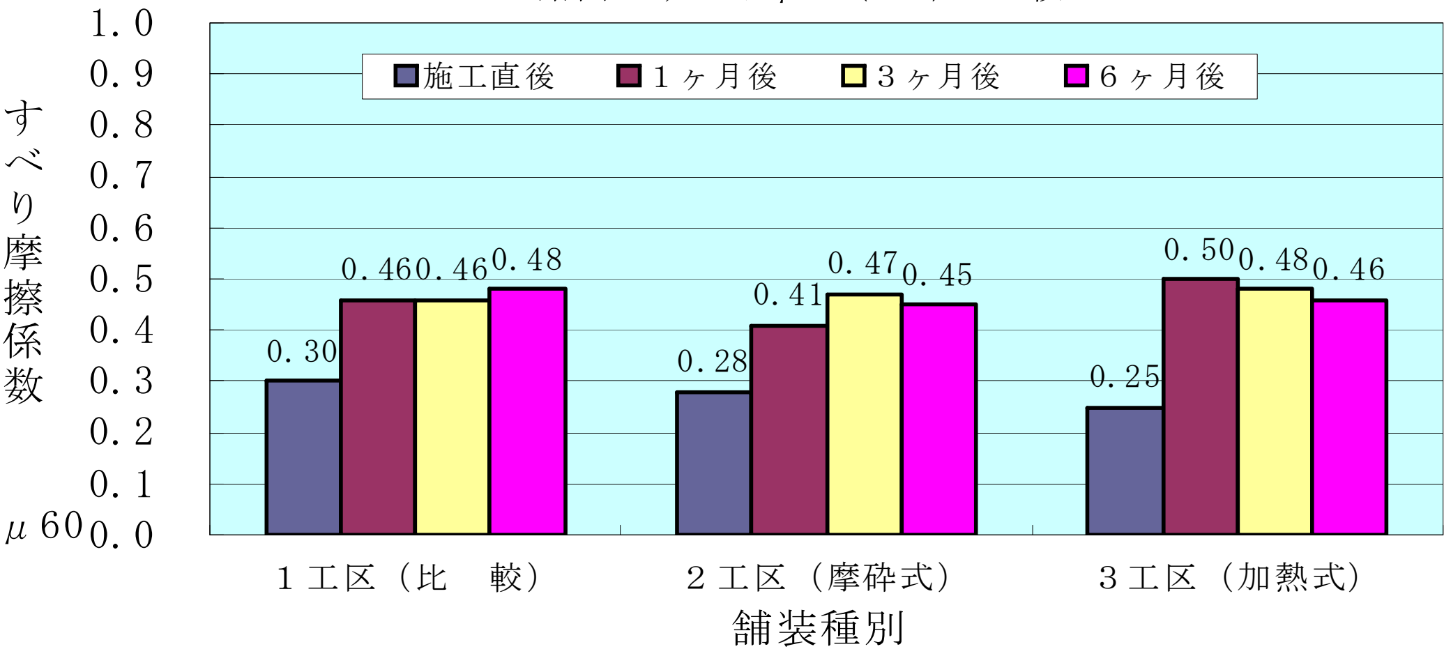
路面のすべり \mu_{60} (IWP) の比較
