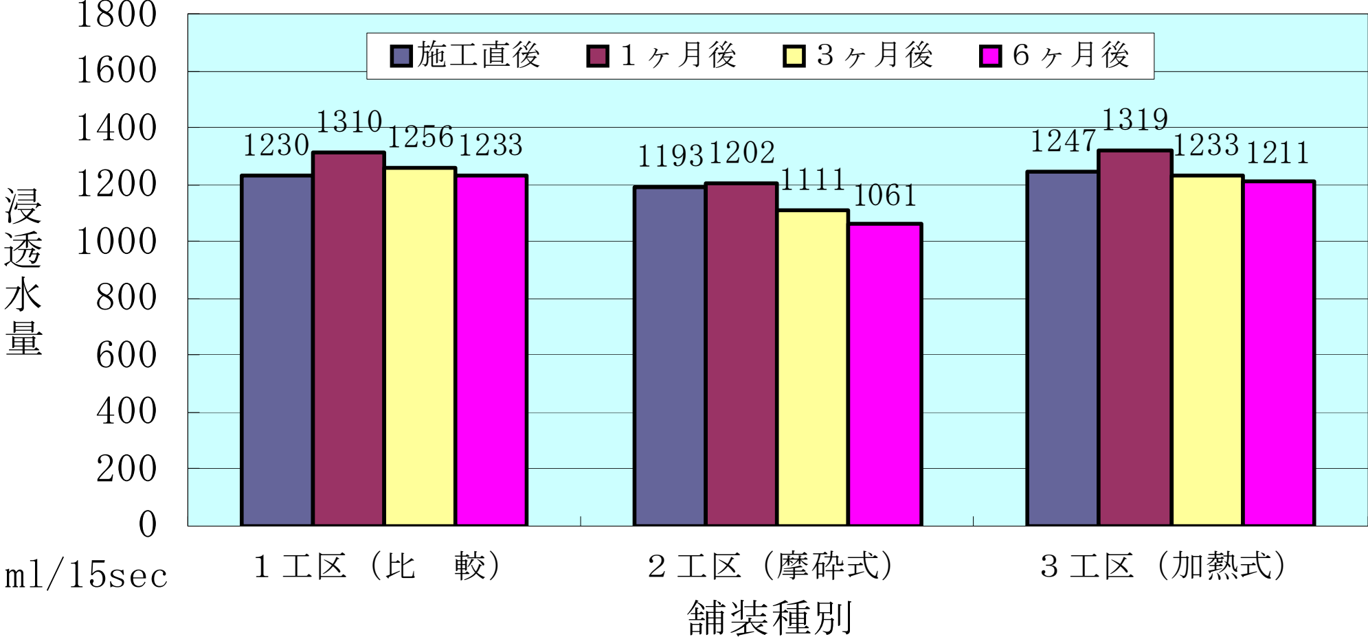
浸透水量(OWP)の比較
