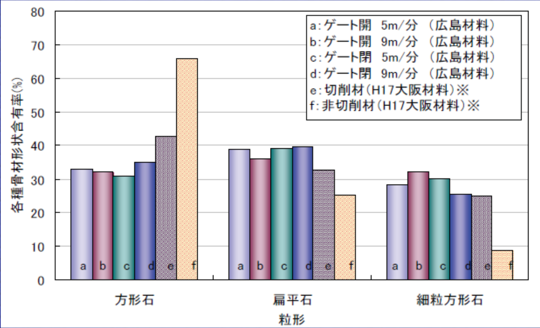
撤去収集方法による骨材形状の相違
