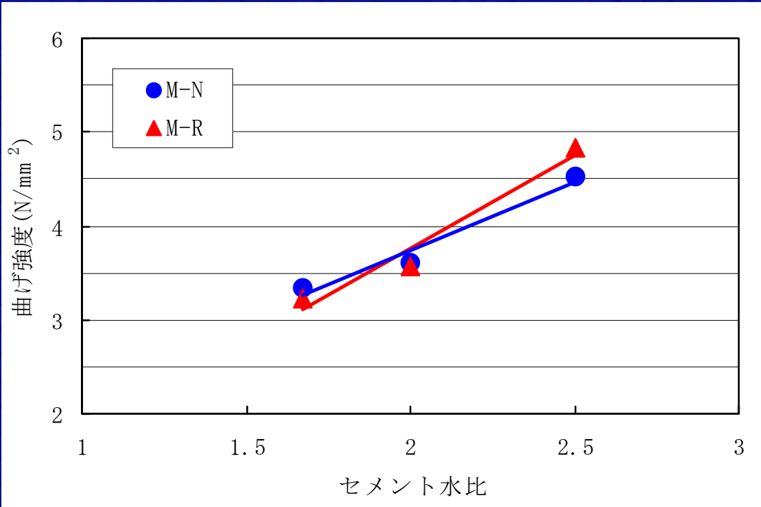
曲げ強度試験結果
