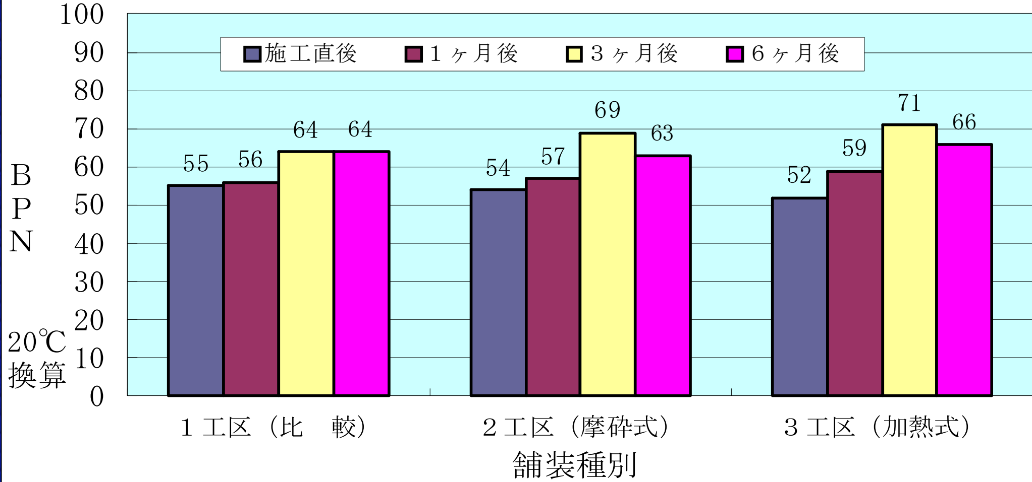
路面のすべり SN (IWP) の比較
