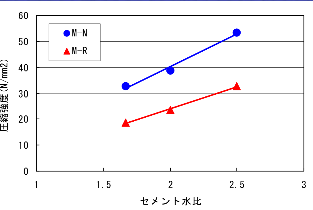
圧縮強度試験結果
