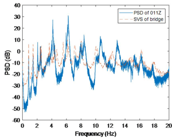
(b) 橋梁部の最短ケーブル振動（C1 ケーブルの 015 センサ）
