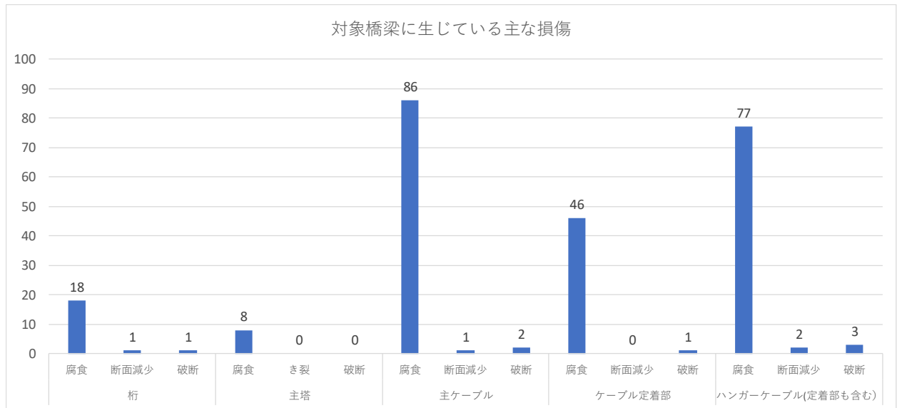
図 2-19 吊り橋に生じている損傷状況
