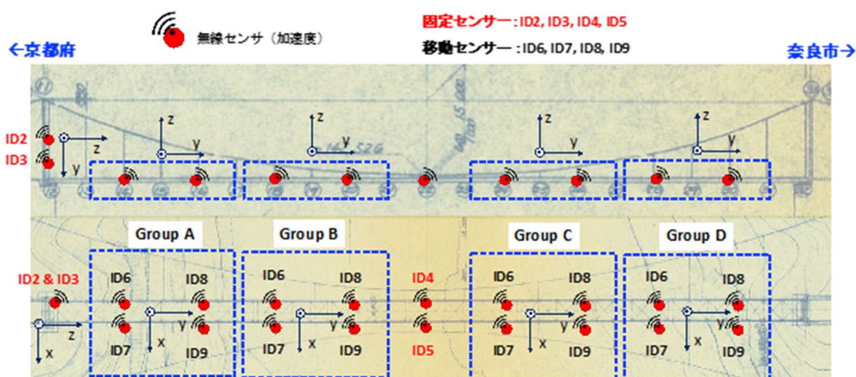
図3-4 センサ・グルーピング・シナリオ1の移動センサグループ
