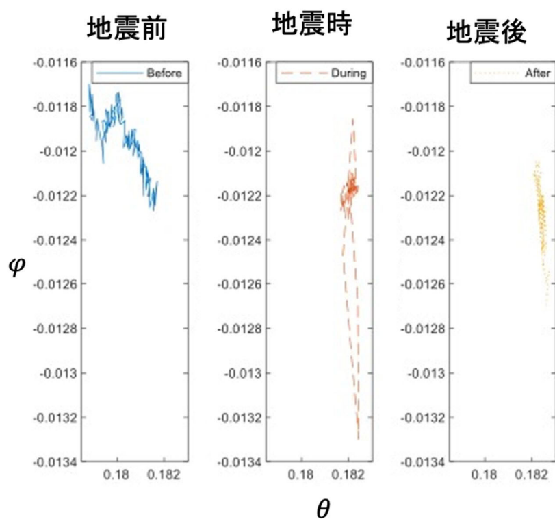
図3-43 主塔の地震前後および地震時の傾斜角の軌道 (INC1, 計測間隔: 1 回/10 秒)
