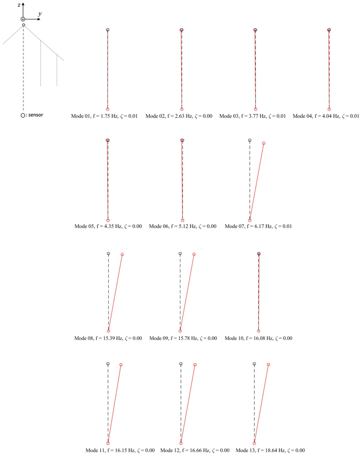
図 3-30 主塔（京都府側）の振動モード（y-z 平面）
