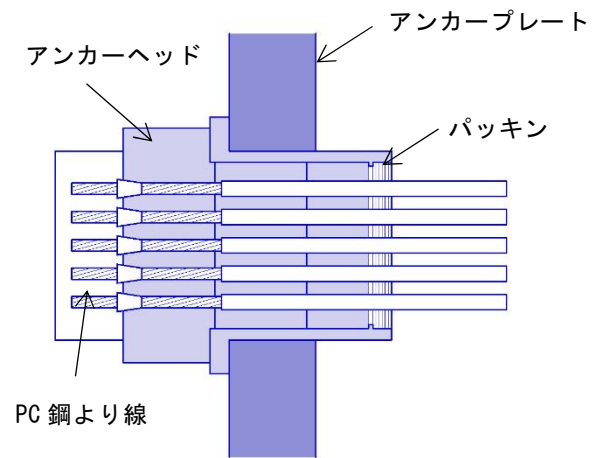
図 2-6 くさび止め定着構造事例
