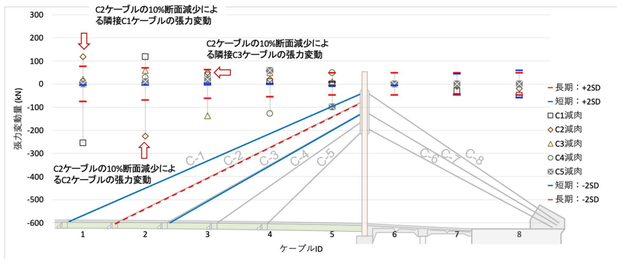
図 4-21 橋梁部ケーブルの断面欠損によるケーブル張力の変化
