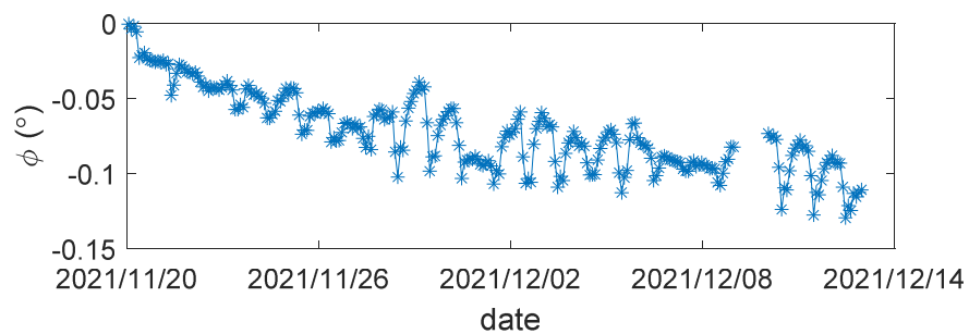
(b) 主塔の傾斜角(INC2 センサ:下流側)
