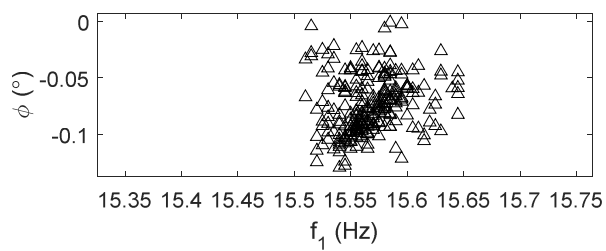
(a) INC1 の回転角と ACC3 の卓越振動数の関係
