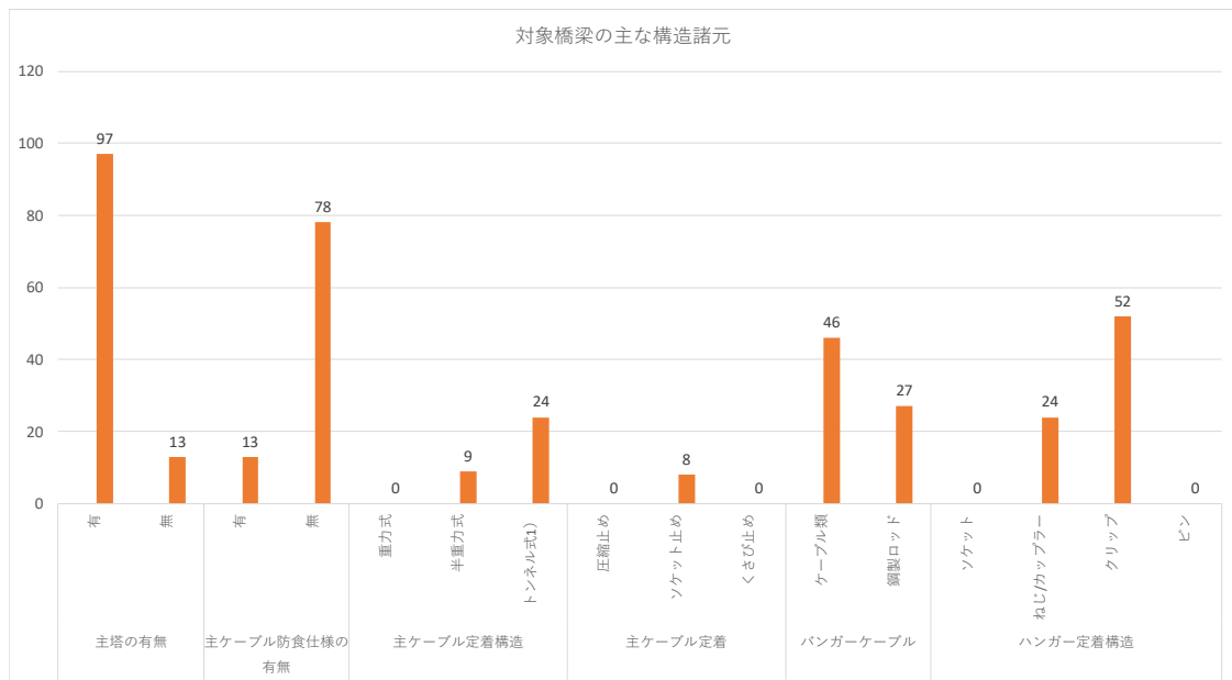
図 2-18 吊り橋の主な構造諸元
