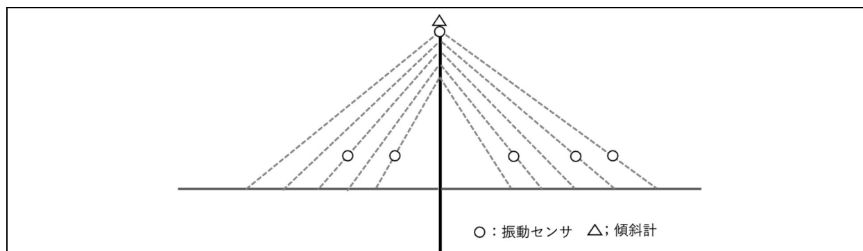
図 5-5 小規模斜張橋の簡易モニタリング：2面吊り方式斜張橋
