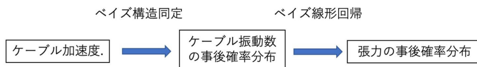
図 5-7 ベイズケーブル張力同定の流れ
