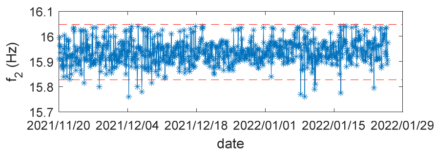
(b) 下流側ケーブル振動(ACC4 センサ)
