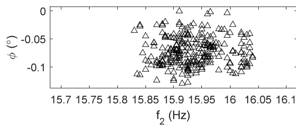
(b) INC2 の回転角と ACC4 の卓越振動数の関係
