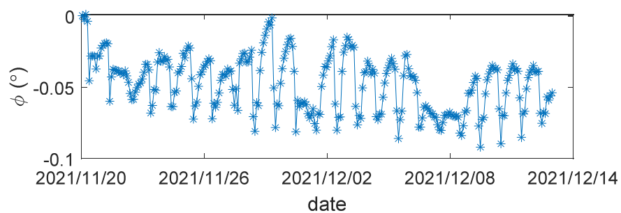
(a) 主塔の傾斜角(INC1 センサ:上流側)
