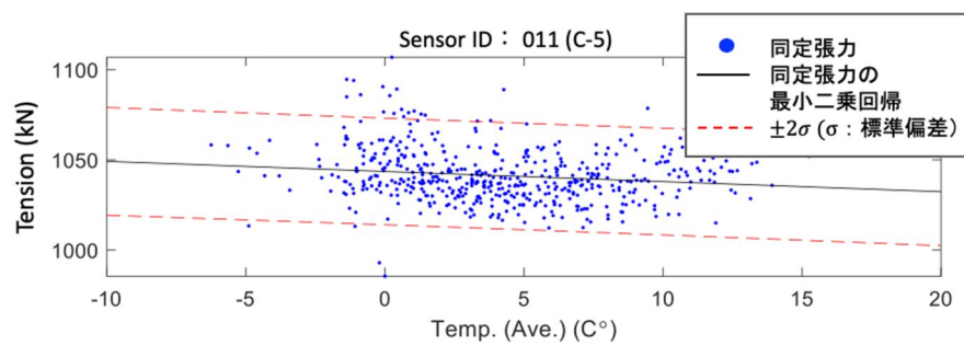
(b) 橋梁部の最短ケーブル
