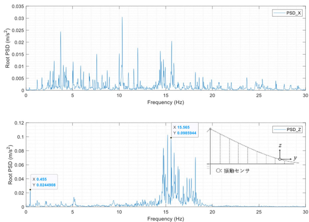
(b) 主ケーブル加速度のPSD (センサ: ACC4)
