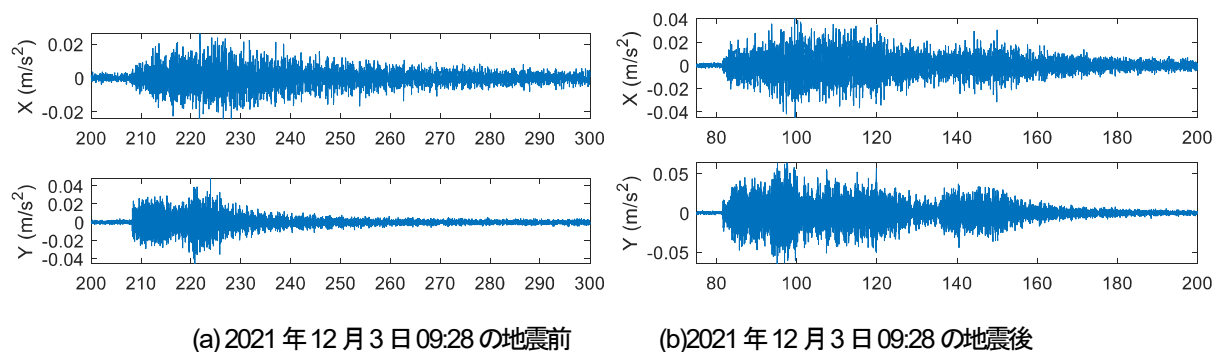
図3-35 主塔の地震前後の加速度時系列 (ACC1) (X: 橋軸直角方向, Y: 橋軸方向)
