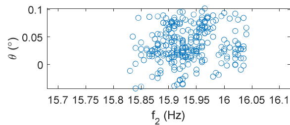
(b) INC2 の傾斜角と ACC4 の卓越振動数の関係
