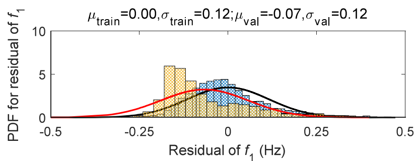
図 B-3 EOV 駆動法による f_1 の予測残差分布（ベイズ線形回帰：BLR）
