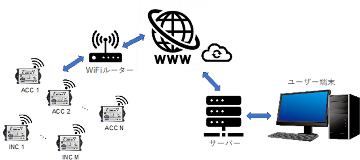
図 3-17 長期モニタリングにおける WiFi 無線センサネットワーク
