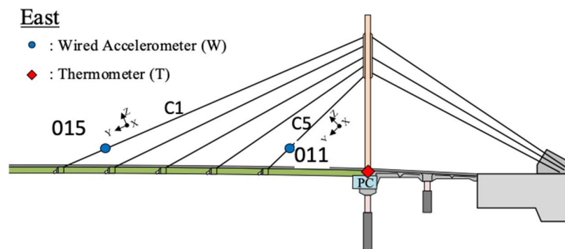
図 4-10 センサ配置（長期モニタリング）
