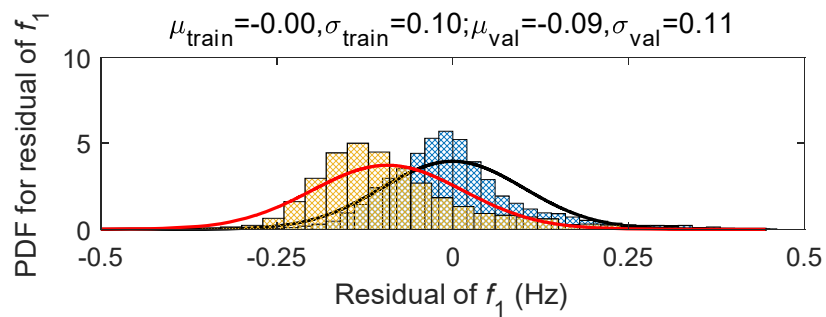
図 B-4 EOV 駆動法による f_1 の予測残差分布（ガウス過程回帰：GPR）
