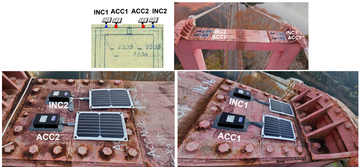
図 3-12 長期モニタリング用の塔頂部の振動センサとソーラーパネル設置状況（INC:傾斜, ACC:加速度）
