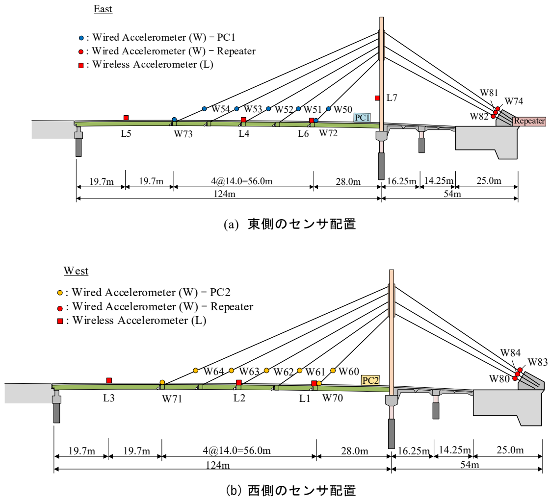
図 4-3 短期モニタリングにおけるセンサ配置
