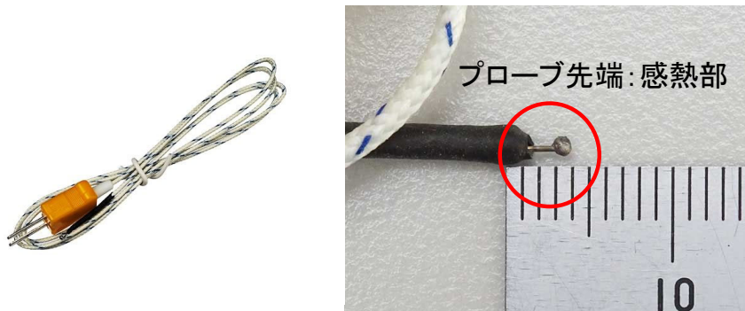
図3-18 長期モニタリングに導入したK型熱電対
