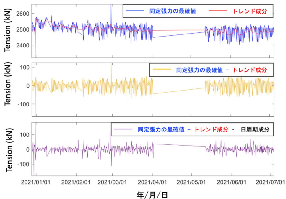
図 5-10 非 E0V 駆動法の特異スペクトル解析による季節変動成分の分離（上段：図 4-13(a)のケーブル張力の最確値（元データ）と SSA より分離した長期トレンド成分，中段：元データに長期トレンド成分を除去した張力の時系列，下段：元データに長期トレンド成分を除去した張力の時系列から日周期成分を除去した張力の時系列）
