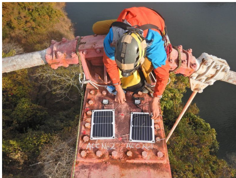
写真 2-6 主塔上での作業状況
