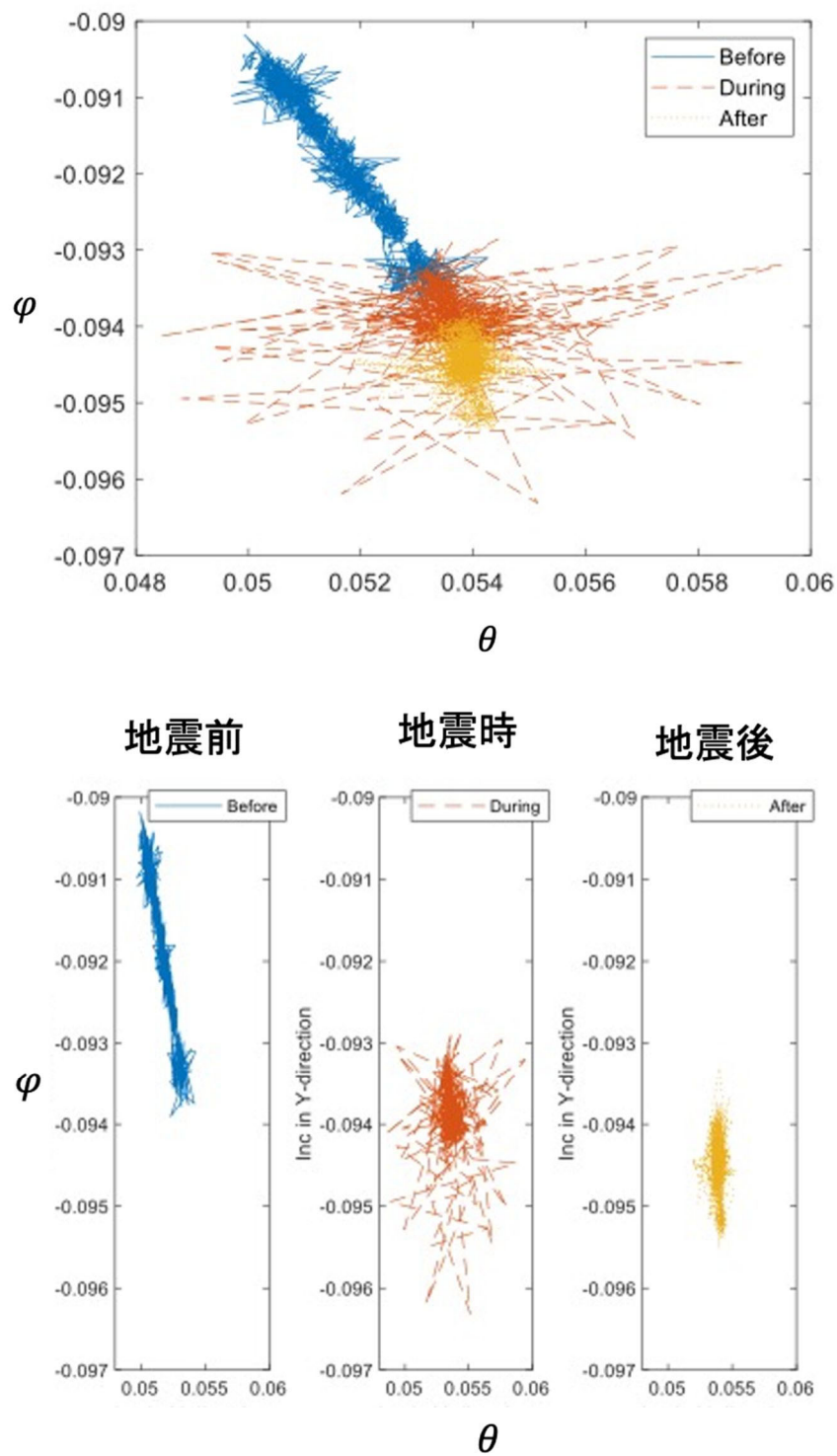
図3-44 主塔の地震前後および地震時の傾斜角の軌道 (INC2, 計測間隔: 1 回/秒)
