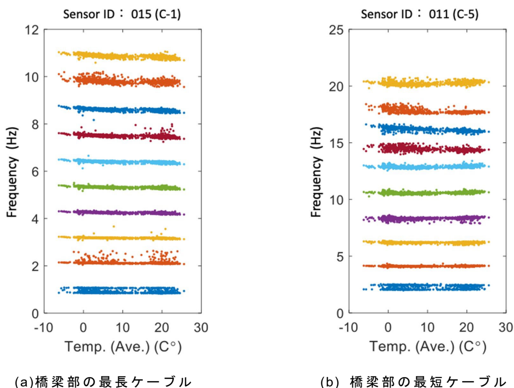
図4-12ケーブル振動数と温度の関係
