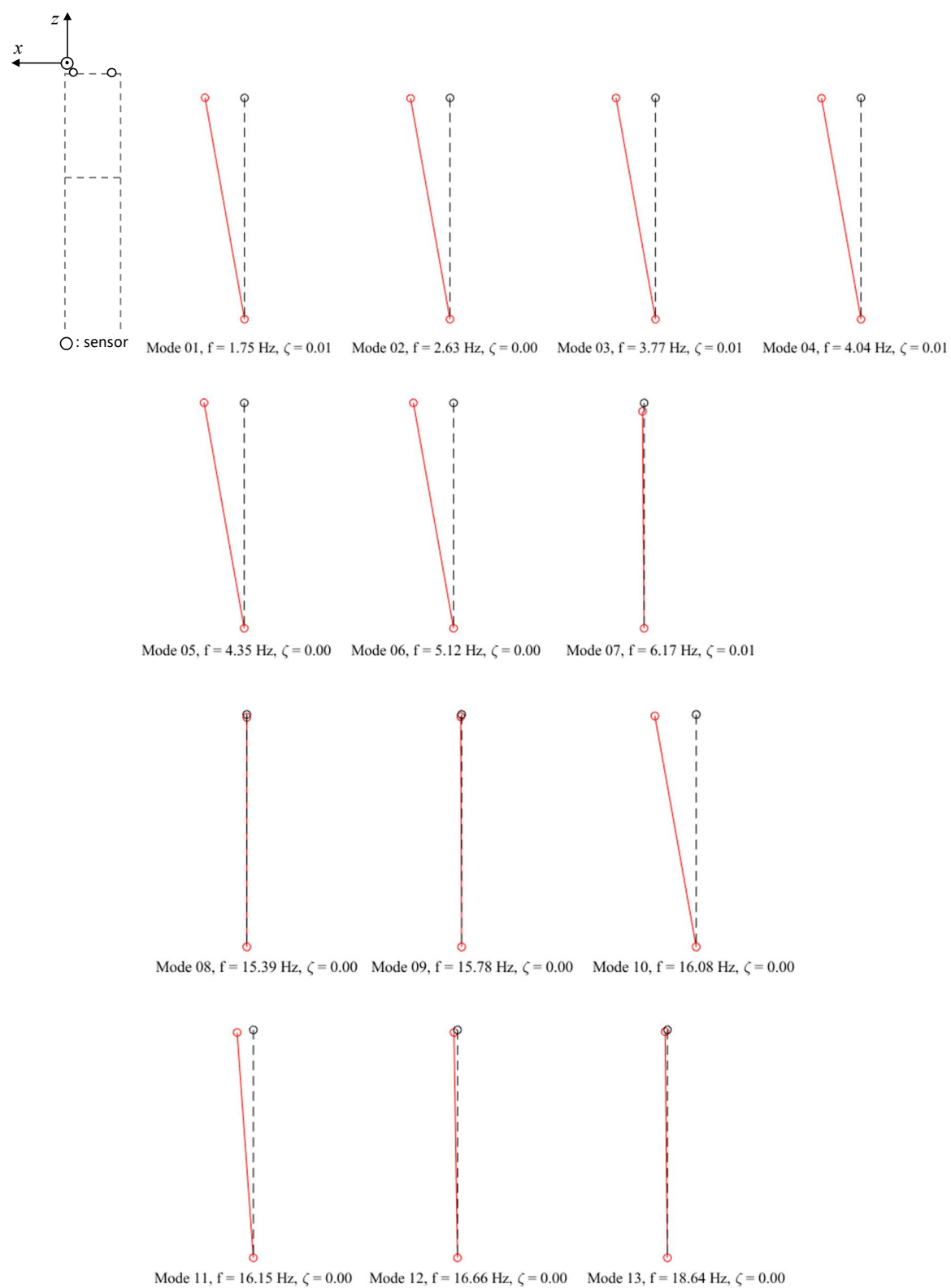
図3-29 主塔（京都府側）の振動モード（x-z 平面）
