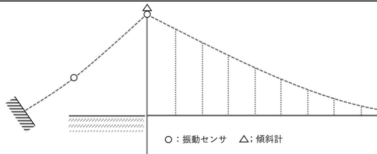
図 5-2 小規模吊り橋の簡易モニタリング：定着部の主ケーブルが複数に分かれていない場合
