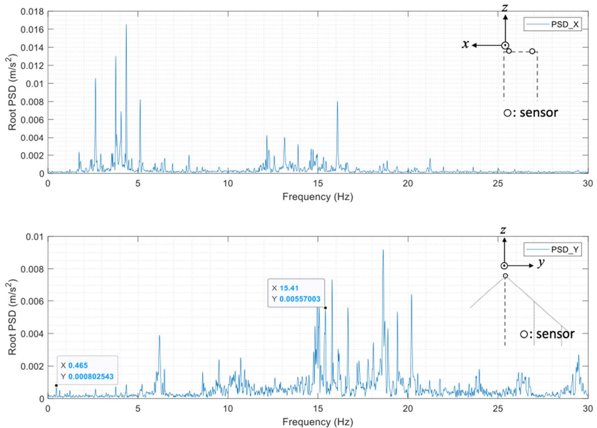
図 3-27 主塔振動の PSD (ACC1 の加速度)
