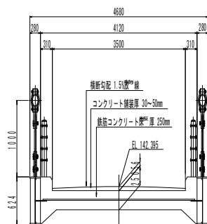
横断面図 S=1:30
