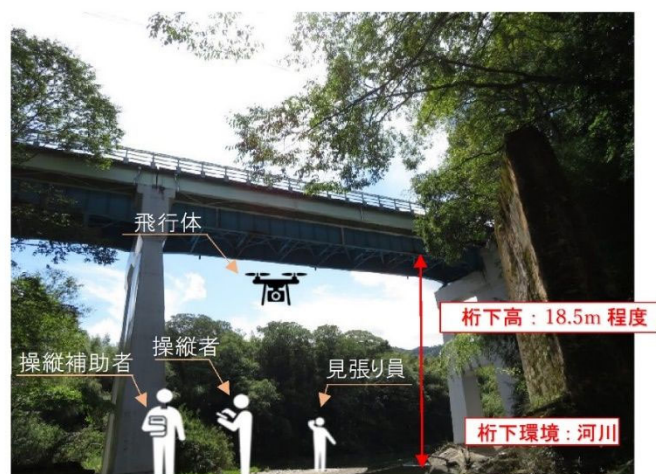
図 2-17 ドローンを用いた点検イメージ図
