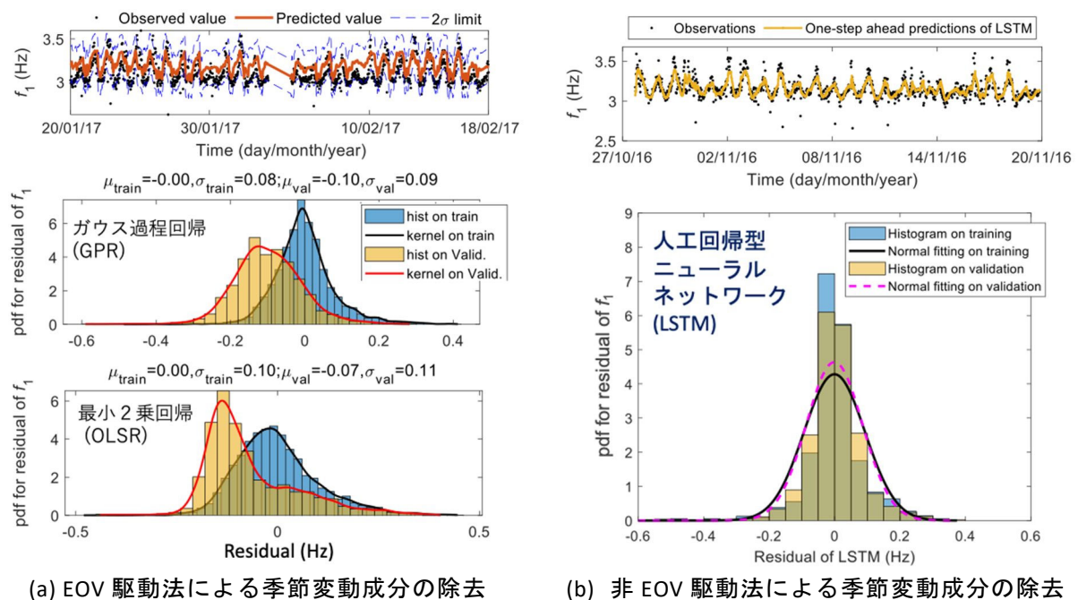
図 5-9 EOV 駆動法と非 EOV 駆動法による季節変動成分の除去後の予測誤差分布
