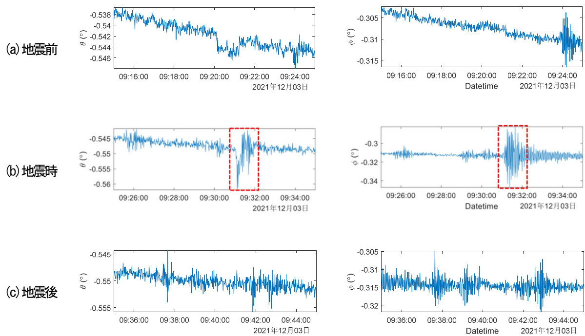
図3-42 主塔の地震前、地震時および地震後の傾斜角と傾斜角（INC2，計測間隔：1回/秒）
