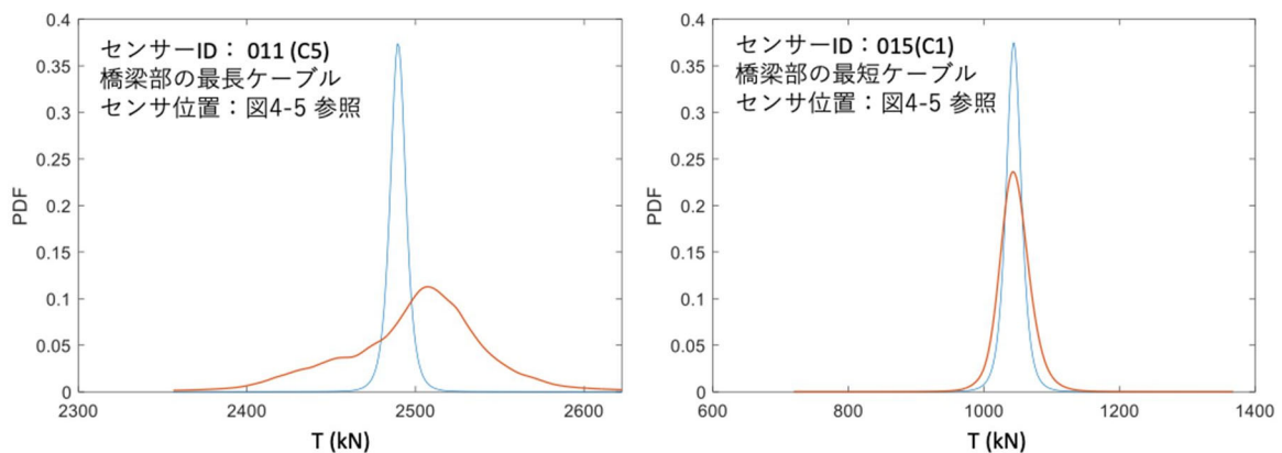
図 5-8 短・長期モニタリングの同定ケーブル張力の事後確率分布（青線：短期計測，赤線：長期計測）
