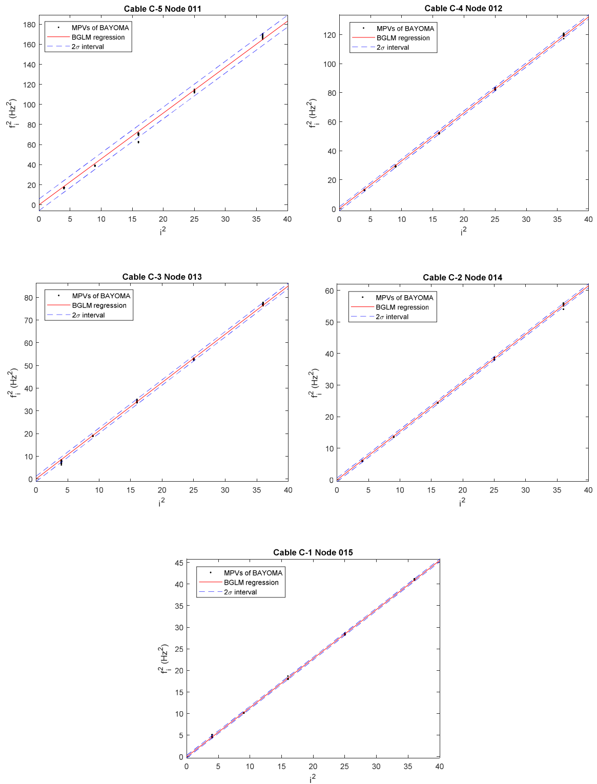
図 4-7 桁部ケーブル振動数と振動次数の線形回帰（黒点：振動数の最確値と振動次数の関係，赤線：ベイズ一般化線形モデル，青破線： \pm 2\sigma （ \sigma ：標準偏差））。
