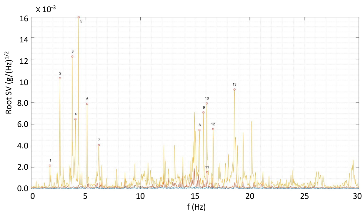
図3-28 主塔（京都府側）振動の平均特異値スペクトル（ACC1 と ACC2 センサ）。
