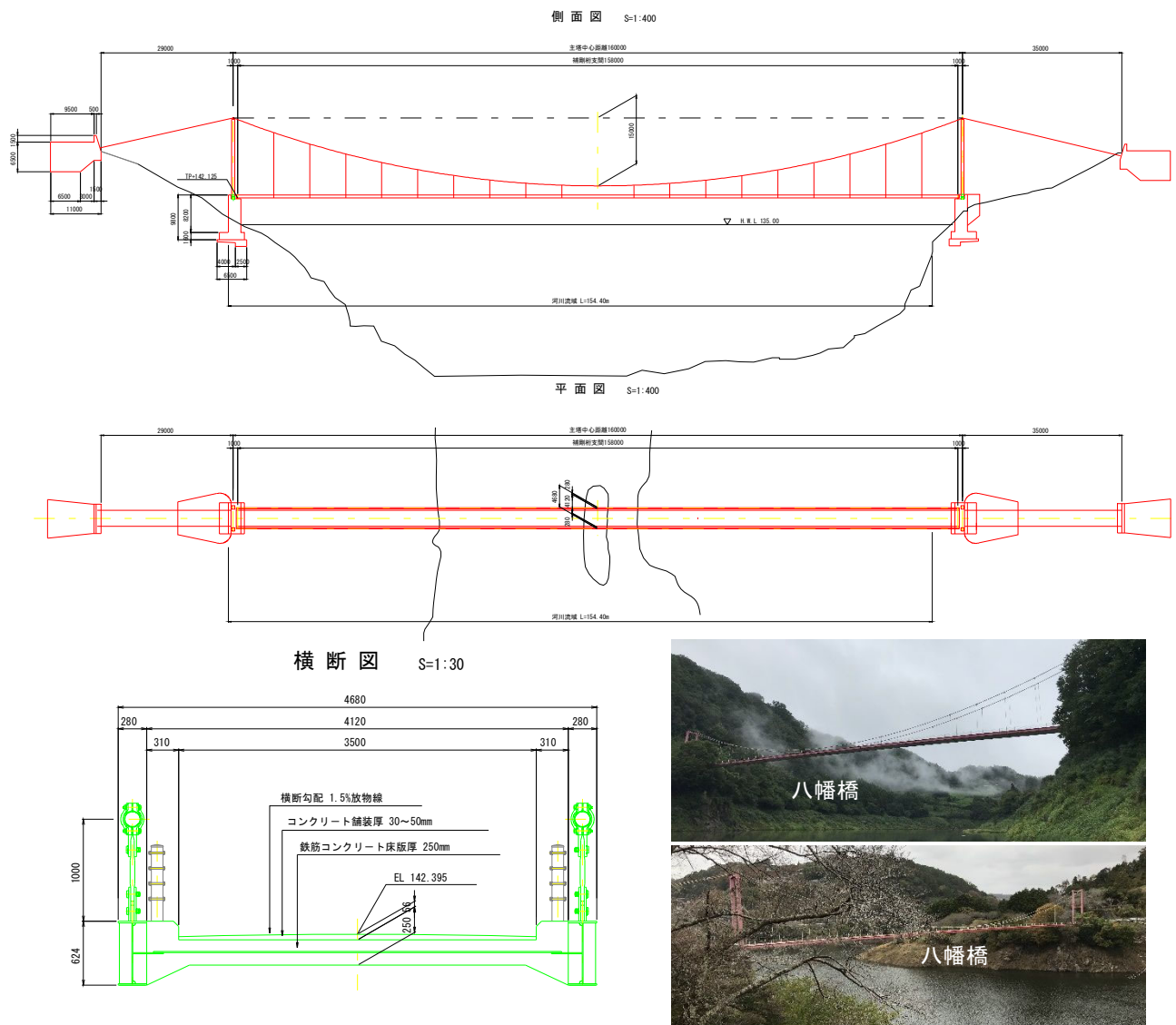
図 2-7 八幡橋概要図
