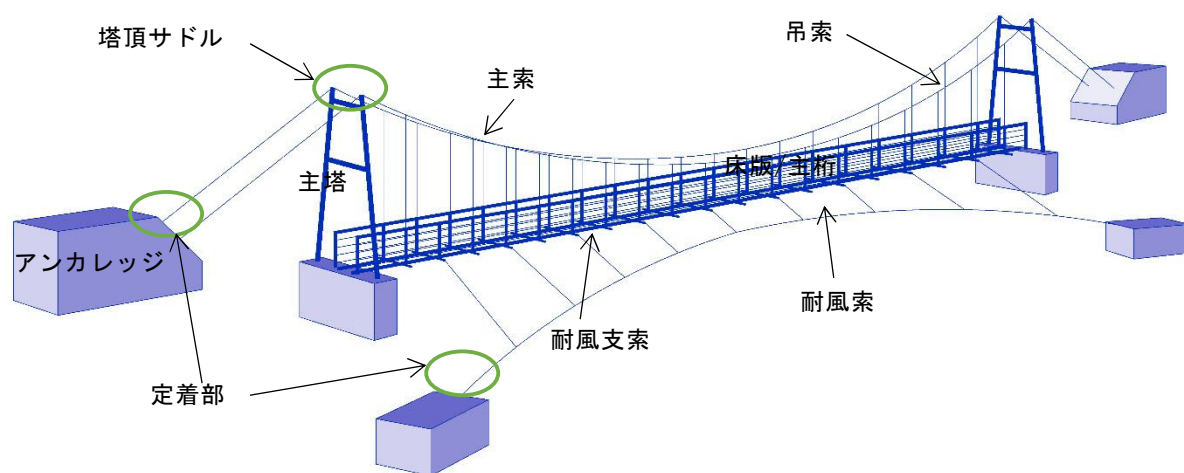
図 2-3 吊り橋構造概要図
