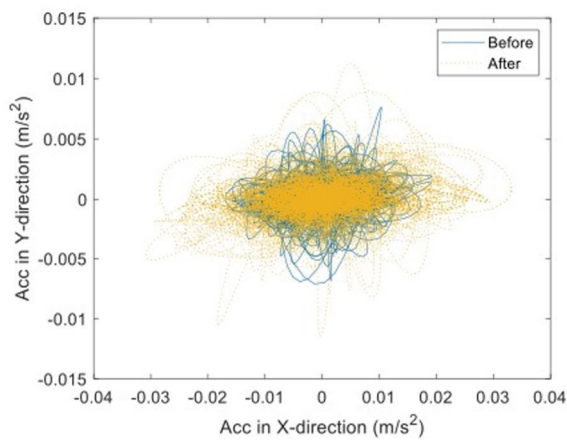
図 3-38 主塔の地震前後の加速度 (ACC1) の軌道 (Before : 地震前, After : 地震後)
