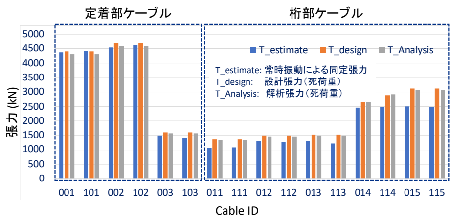
図 4-9 平均同定ケーブル張力，設計張力と解析張力
