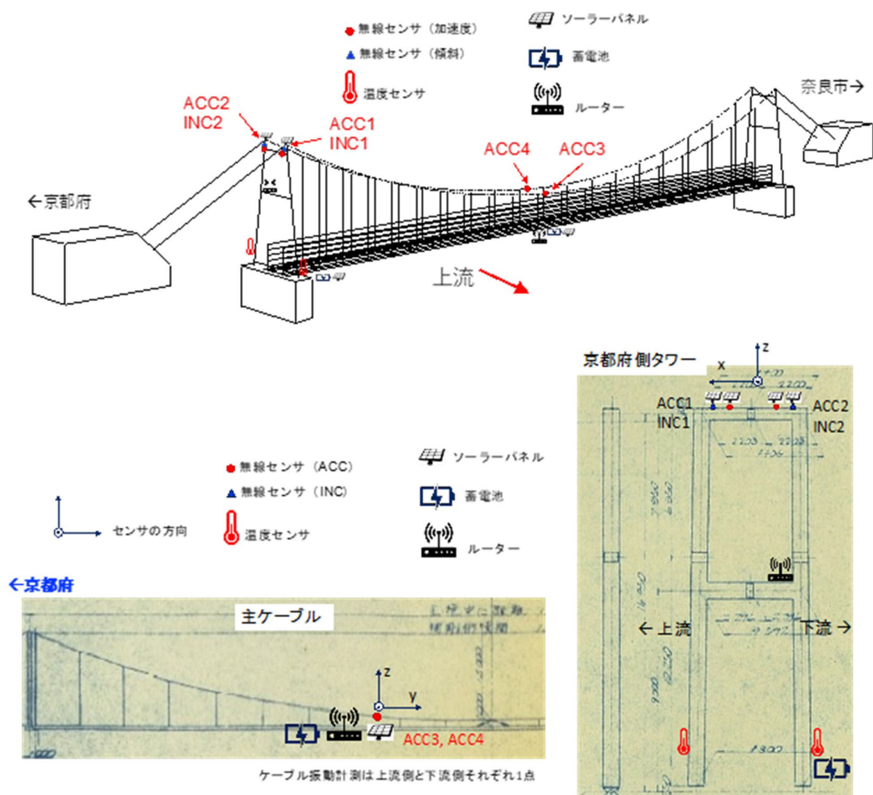
図 3-10 長期モニタリングのセンサと関連機器の配置概要
