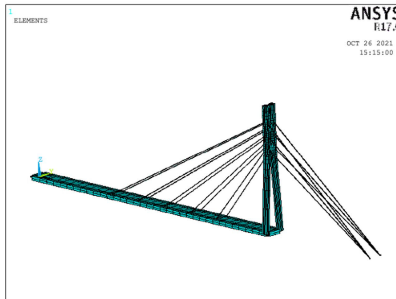
図 4-17 対象斜張橋の有限要素モデル。
