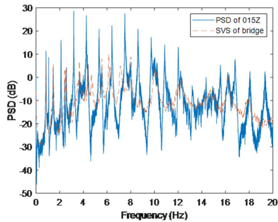
(a) 橋梁部の最長ケーブル振動（C1 ケーブルの 015 センサ）
