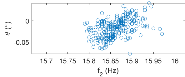
(a) INC1 の傾斜角と ACC3 の卓越振動数の関係
