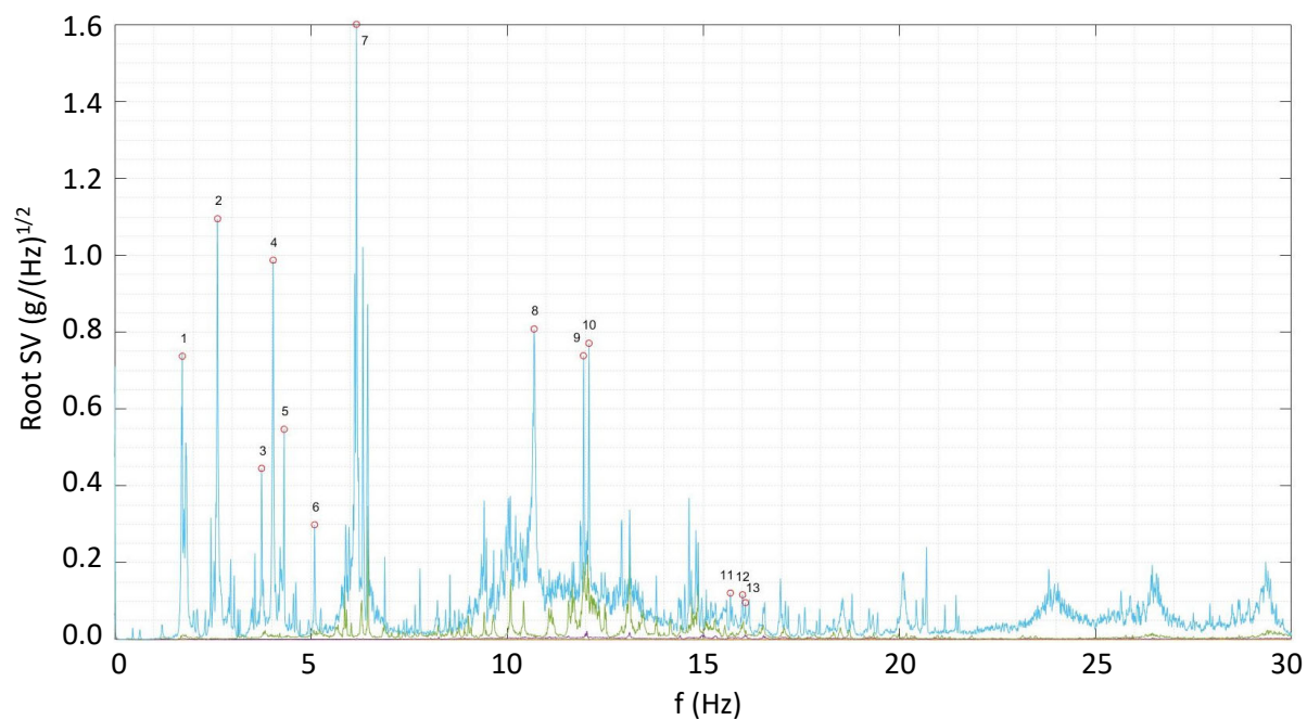
図3-22 主塔（京都府側）振動の平均特異値スペクトル（ID2とID3センサ）。
