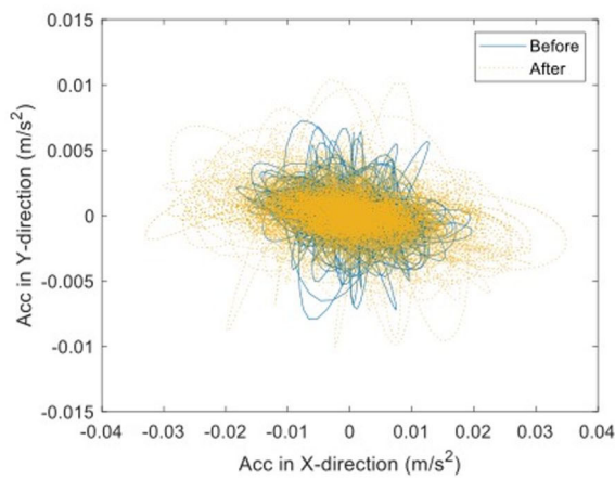
図 3-39 主塔の地震前後の加速度 (ACC2) の軌道 (Before : 地震前, After : 地震後)
