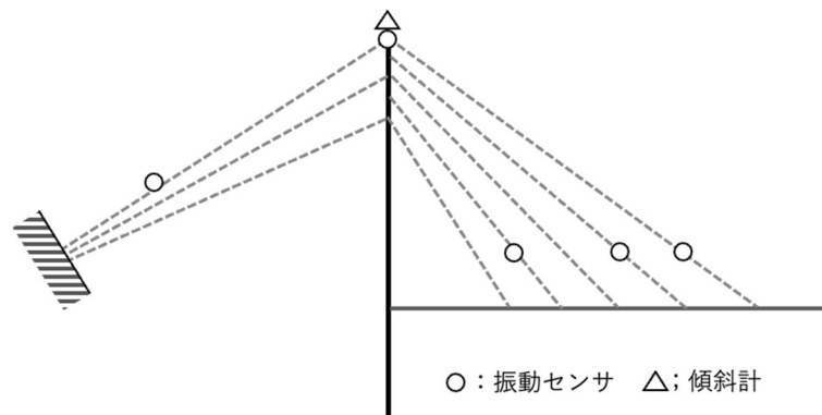
図 5-6 小規模斜張橋の簡易モニタリング：片持ち式斜張橋
