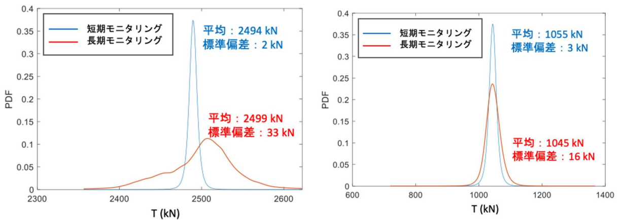
(a) 橋梁部の最長ケーブル (長期モニタリングの同定張力の分布は正規分布ではなく右に偏っていることに注意)
