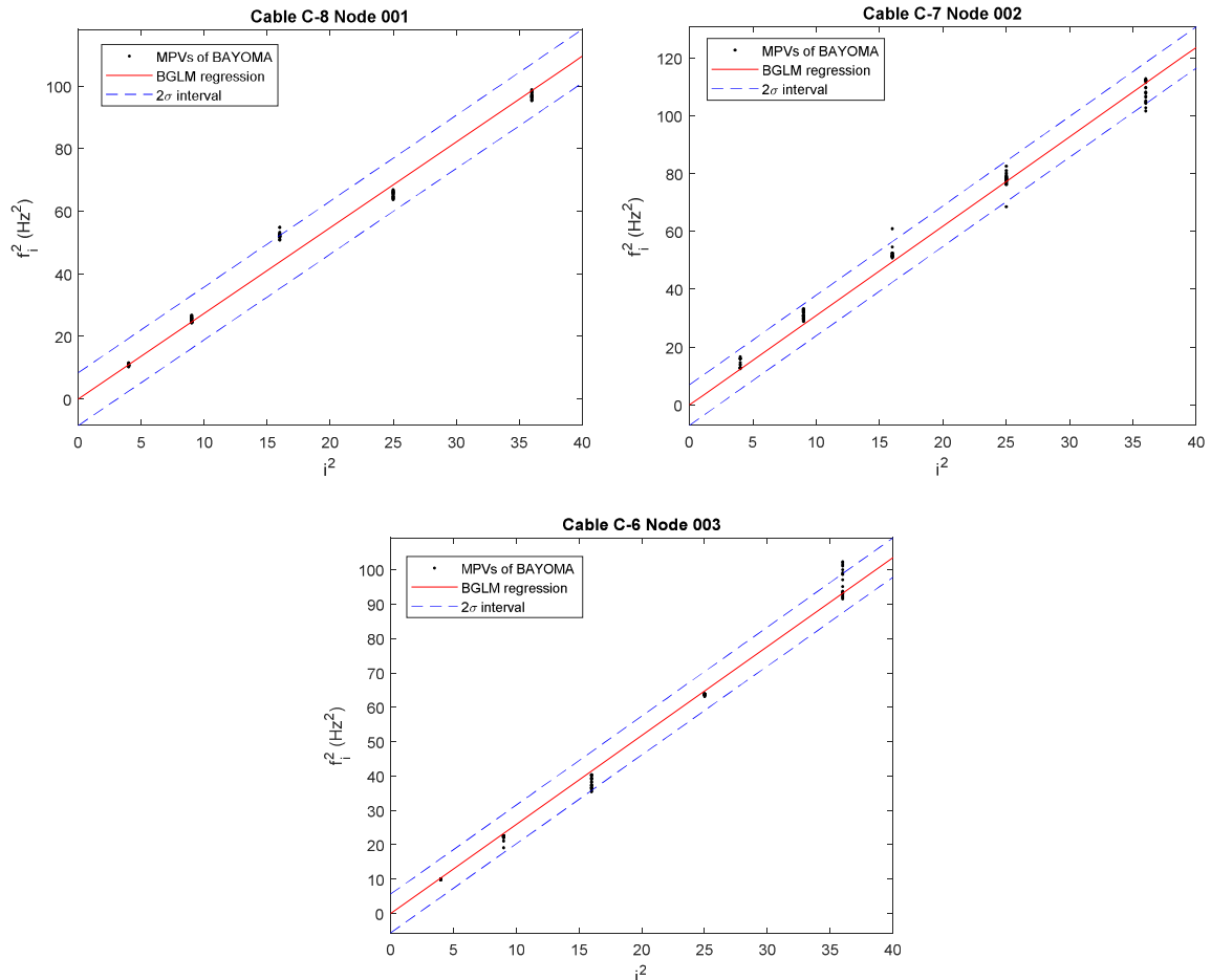
図 4-8 定着部ケーブル振動数と振動次数の線形回帰（黒点：振動数の最確値と振動次数の関係，赤線：ベイズ一般化線形モデル，青破線： \pm 2\sigma （ \sigma ：標準偏差））。
