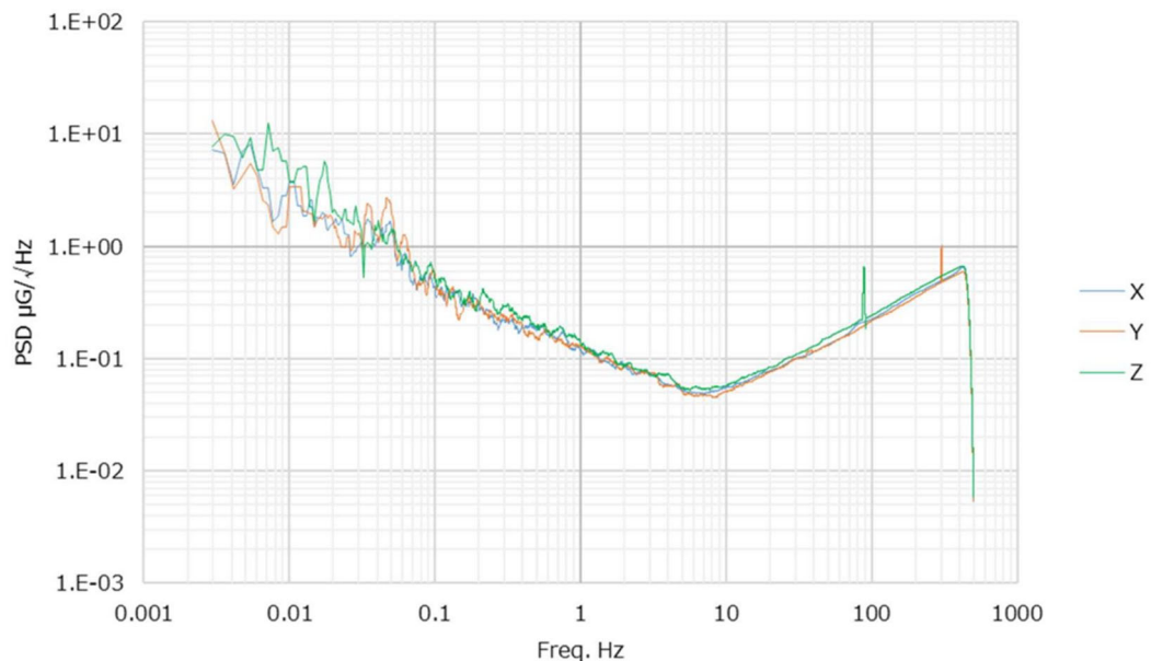
図 3-8 モニタリングに導入した加速度センサの自己雑音のパワースペクトル密度
