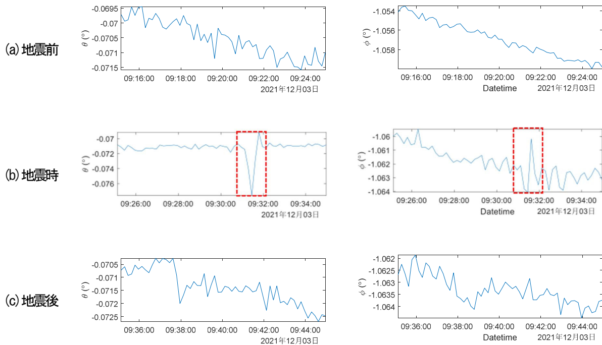
図3-41 主塔の地震前、地震時および地震後の傾斜角と回転角（INC1，計測間隔：1回/10秒）
