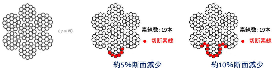
図4-20 断面減少率の計算例に用いたケーブル断面
