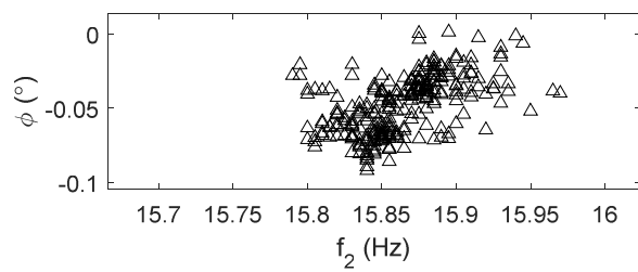
(a) INC1 の回転角と ACC3 の卓越振動数の関係
