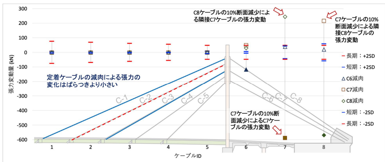
図 4-22 定着部ケーブルの断面欠損によるケーブル張力の変化
