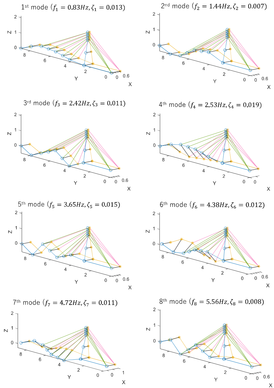
図 4-5 橋梁部振動計測データから同定される平均振動特性
