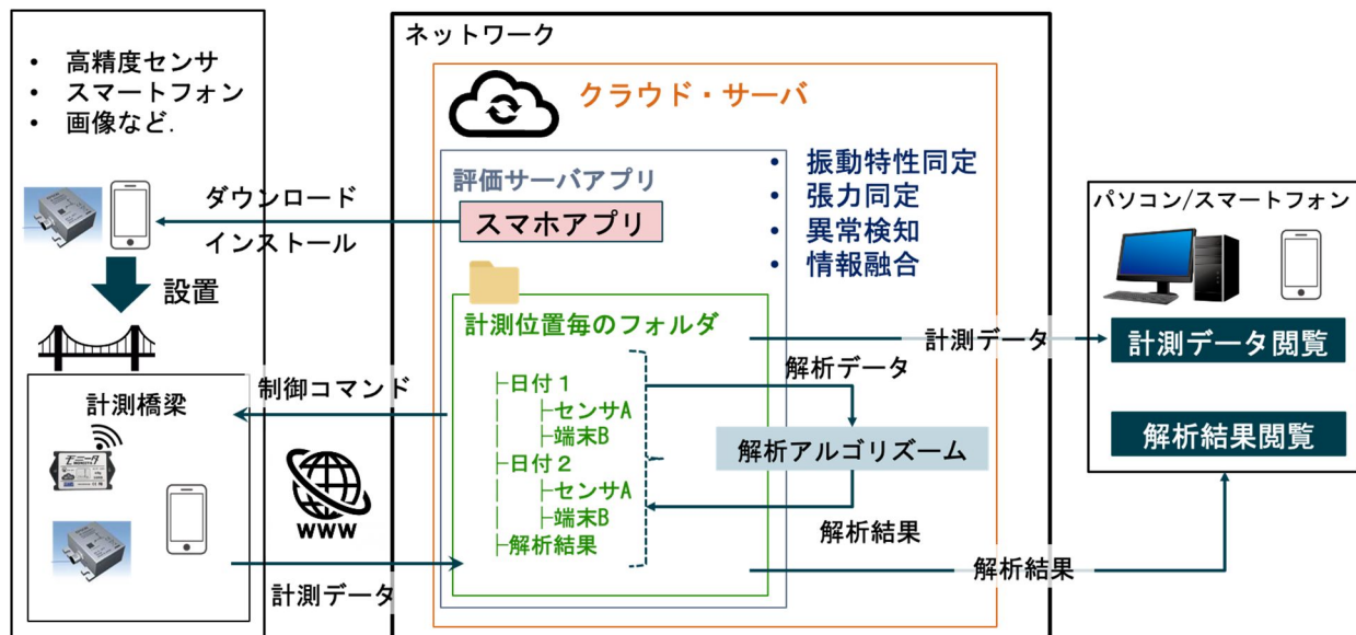
図 5-10 スペククラウド上に運用される長期モニタリングシステムの例
