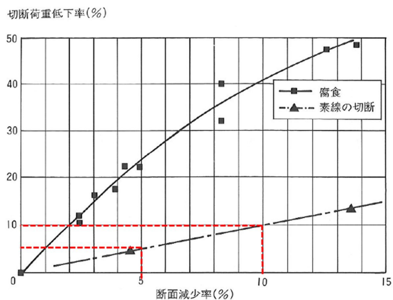
図4-19 断面減少率と切断荷重低下率との関係（野村ら：腐食の生じたストランドロープの残存強度，川田技報，Vol.12, pp.127-130, 1993）
