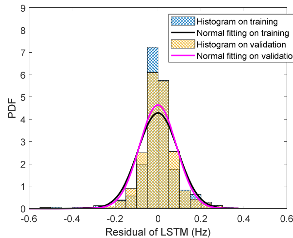
図 B-6 LSTM による f_1 の訓練データと検証データの予測残差分布
