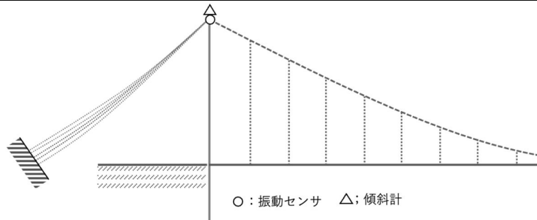
図 5-3 小規模吊り橋の簡易モニタリング：定着部の主ケーブルが複数に分かれている場合
