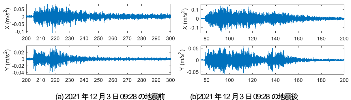
図3-36 主塔の地震前後の加速度時系列 (ACC2) (X: 橋軸直角方向, Y: 橋軸方向)
