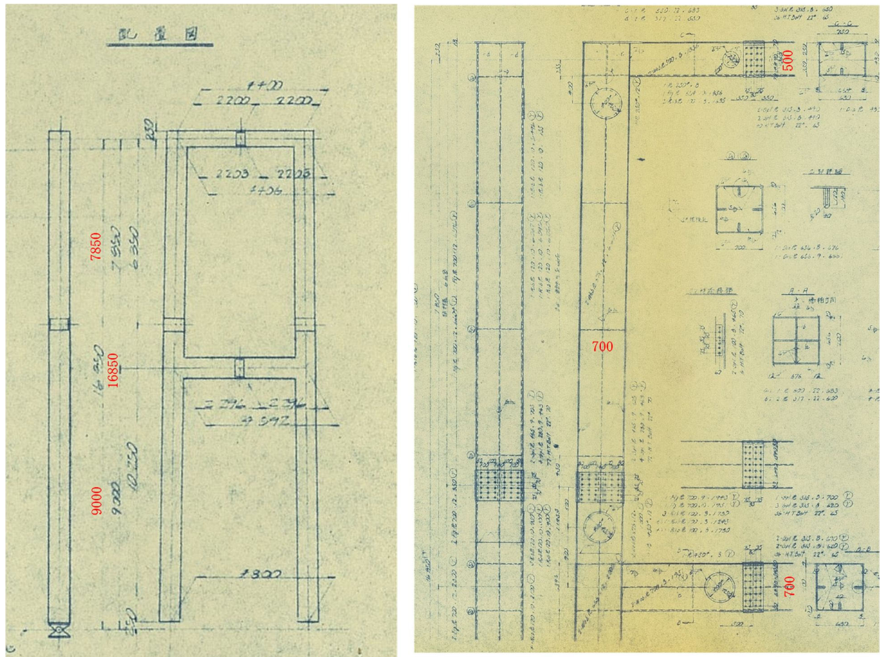
図 2-16 主塔構造図
