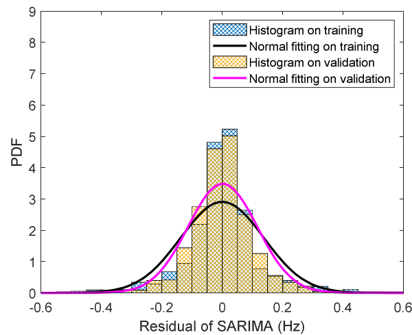
図 B-5 SARIMA モデルによる f_1 の訓練データと検証データの予測残差分布
