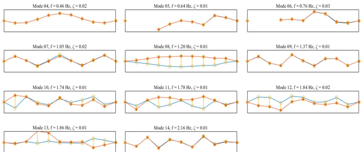
図3-21 桁の鉛直振動モード
