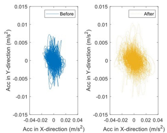
図 3-39 主塔の地震前後の加速度 (ACC2) の軌道 (Before : 地震前, After : 地震後)
