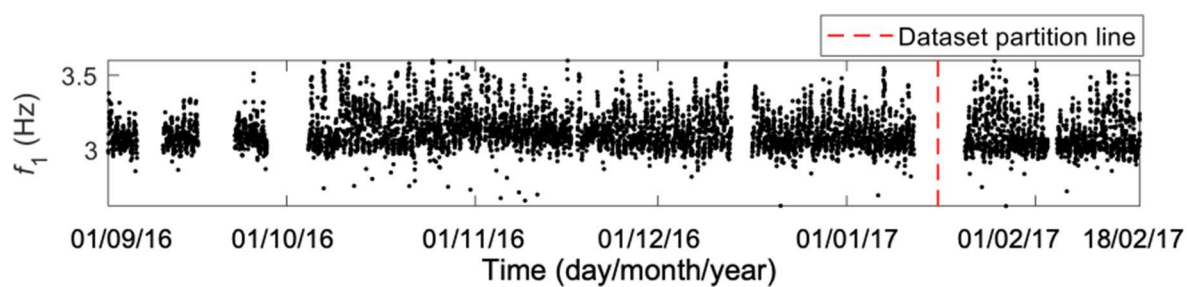
図 B-2 長期モニタリングで観測された振動数の時系列
