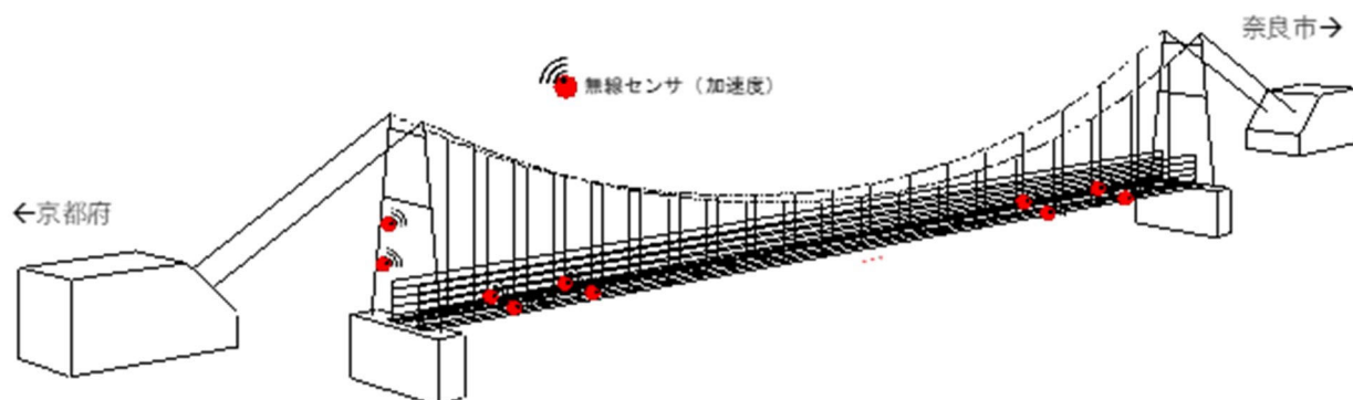
図 3-3 短期モニタリングのセンサ配置概要
