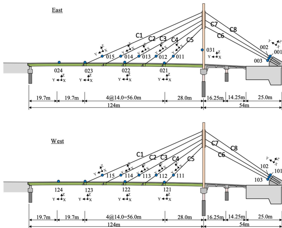
図 4-4 各センサの ID 番号とケーブル ID.
