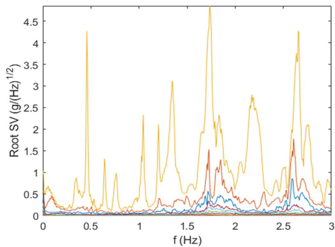
図3-20 Group A ~Group D の平均特異値スペクトル。
