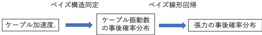
図C-1 ベイズケーブル張力同定の流れ
