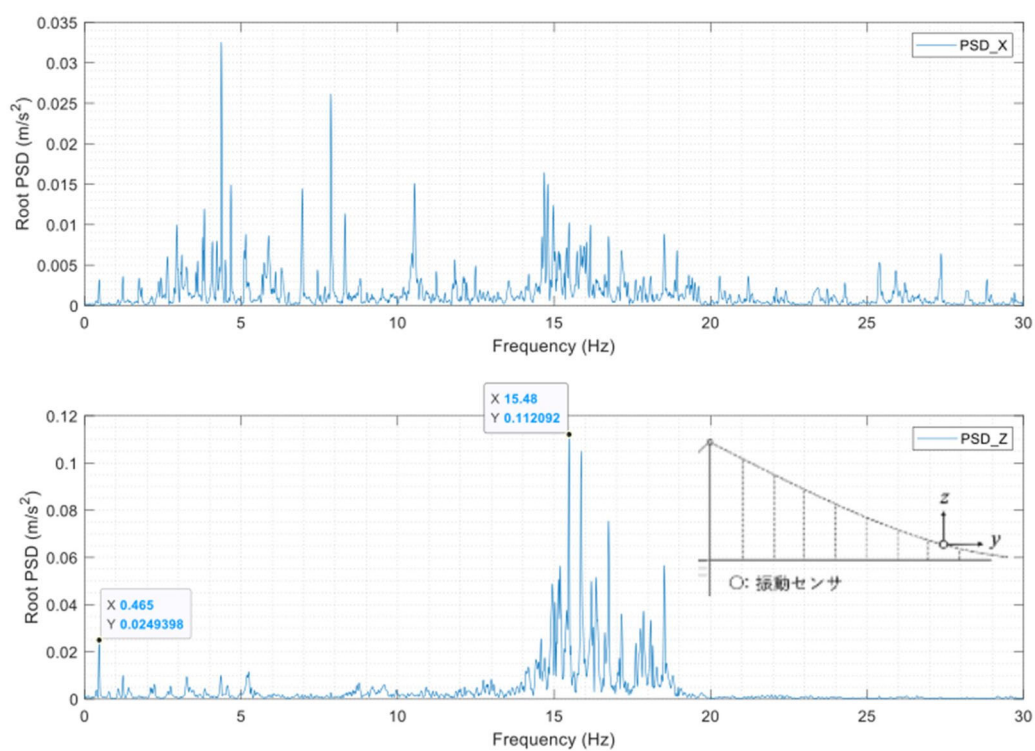
(a) 主ケーブル加速度のPSD (センサ: ACC3)
