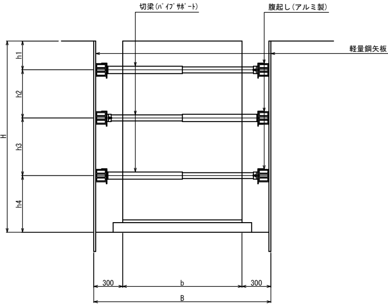
断面図
