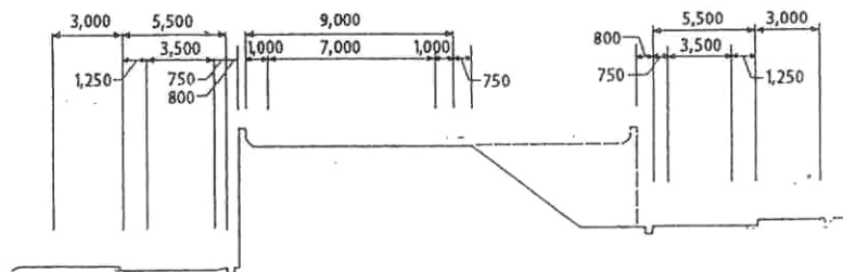
標準断面図
