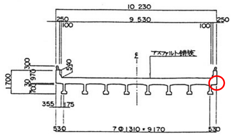
断面图 1:100
