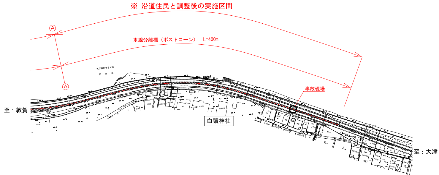
車線分離標 (ポストコーン) (φ80 H650 貼付式)
