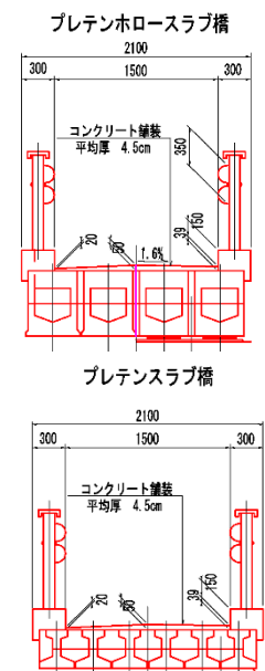
<上部工断面図>
