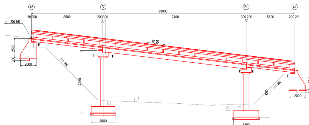
<上部工側面図>
