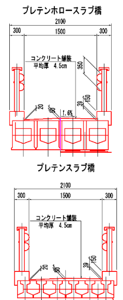
<上部工断面図>
