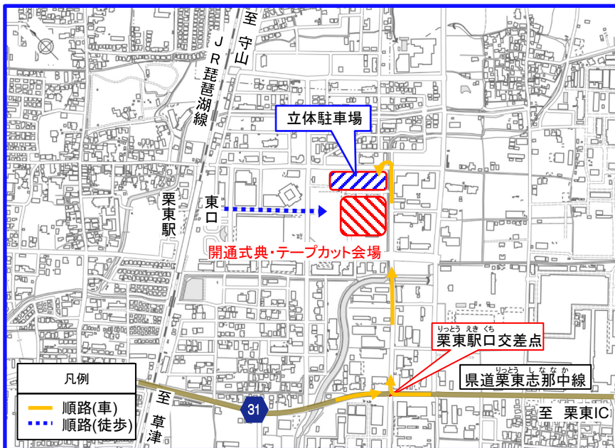
詳細図①
