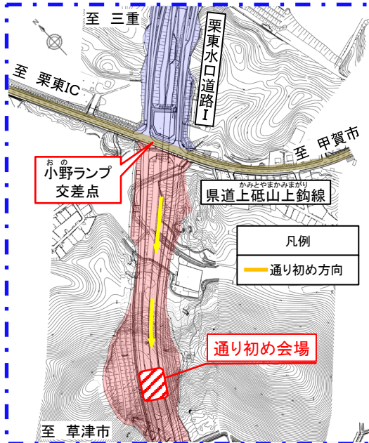
詳細図②
