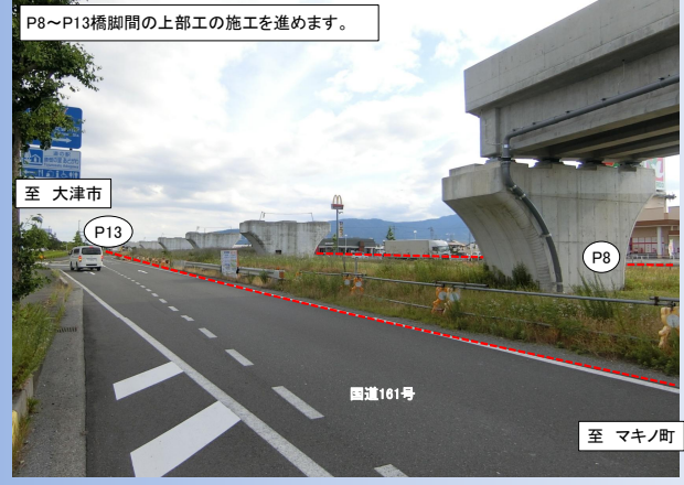
TOPICS 3 国道161号西万木高架橋(P8-P13)PC上部工事 R8.6月 撮影
