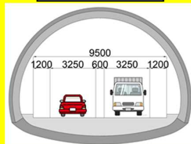
標準断面図
