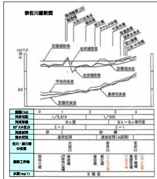
奈佐川縦断面情報図 (直轄区間)
