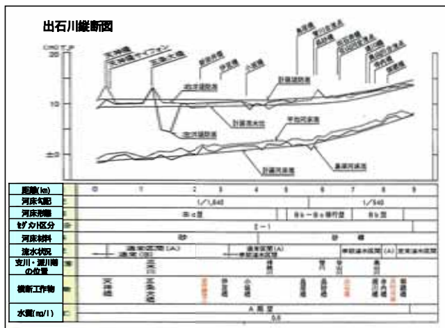
出石川縦断面情報図 (直轄区間)
