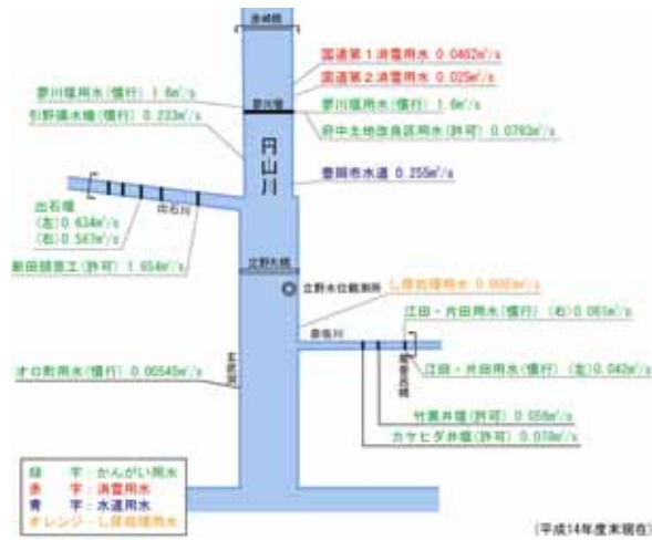
図 水利権モード図
