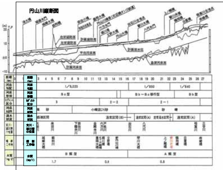
円山川縦断面情報図 (直轄区間)
