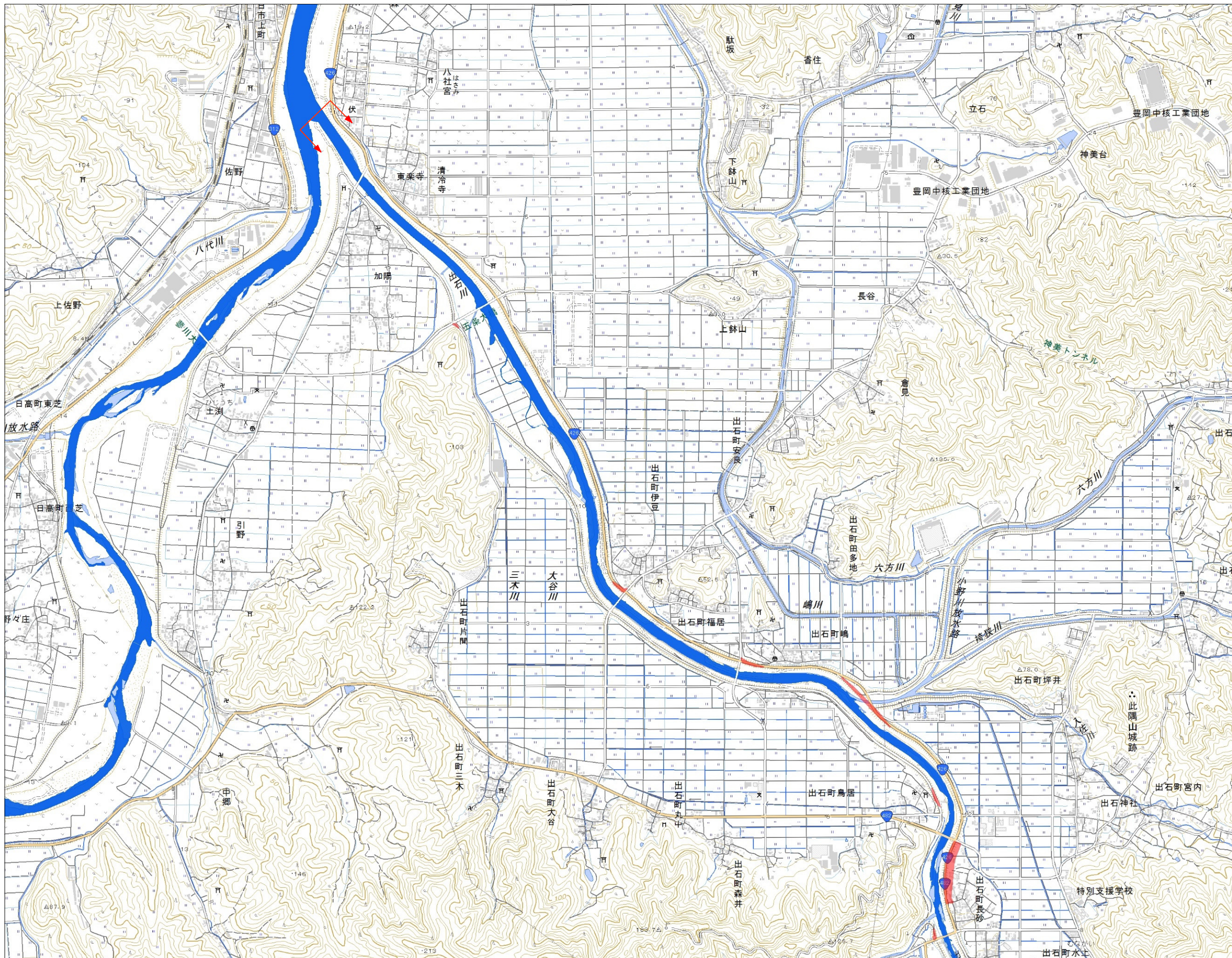
円山川水系出石川洪水浸水想定区域図（家屋倒壊等氾濫想定区域（河岸侵食））（2/3）
