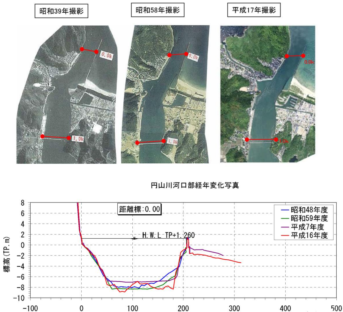
図 1.15 円山川河口部の河道形状の経年変化
