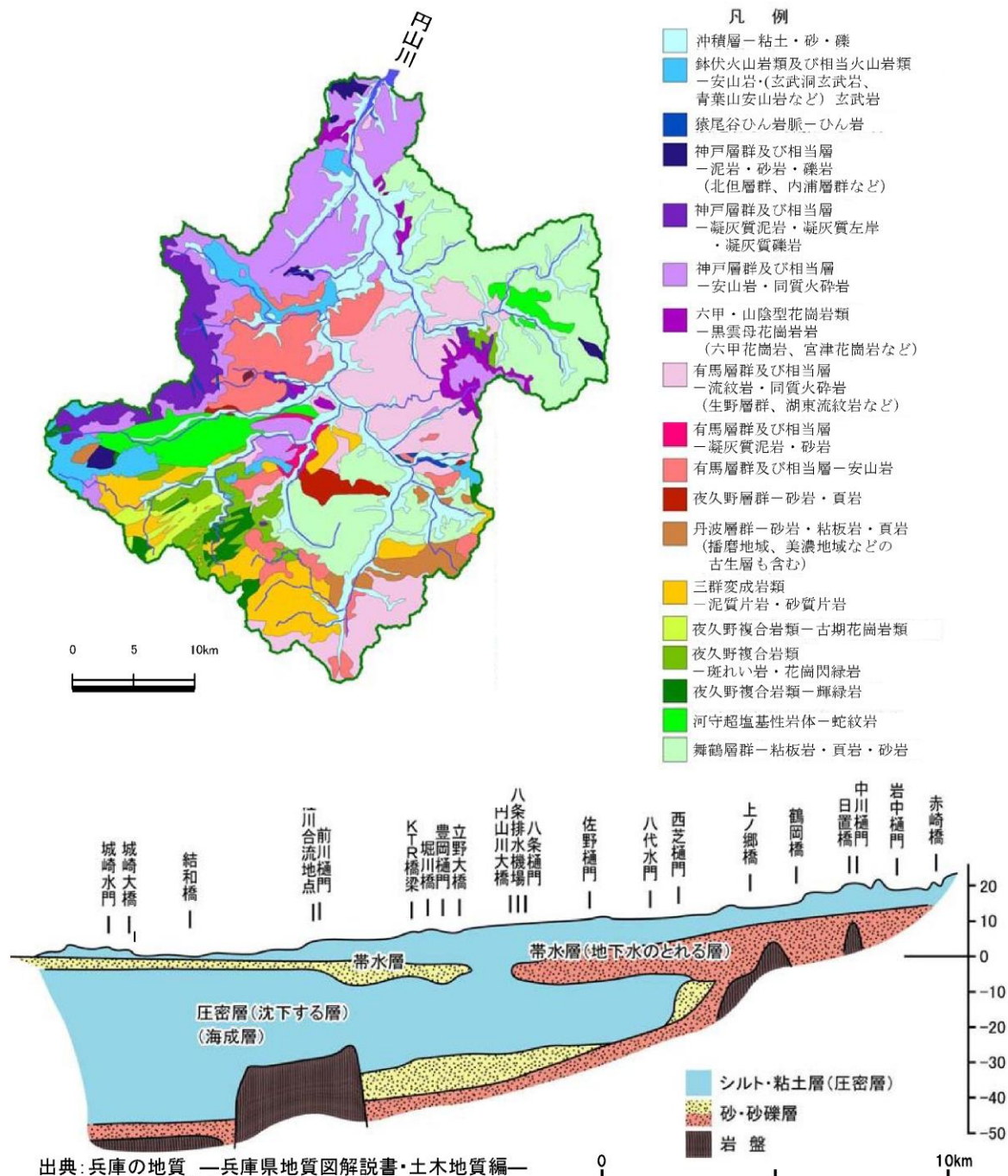
図 1.6 円山川流域地質図(上: 流域の表層地質図、下: 豊岡盆地地質断面図)
