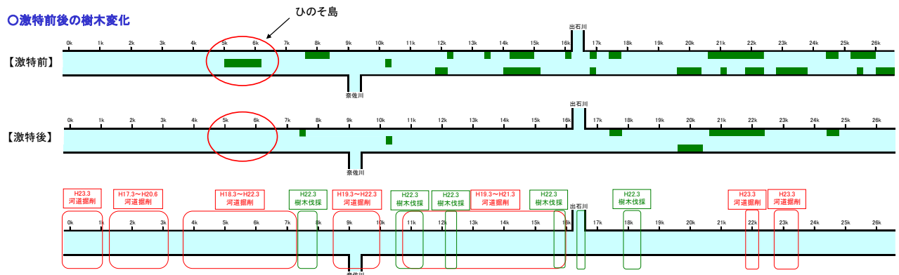
図 1.14 流下阻害となる河道内樹木の伐採状況
