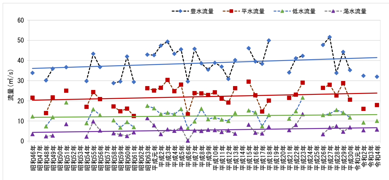
図 1.21 流況経年変化（府市場地点）
