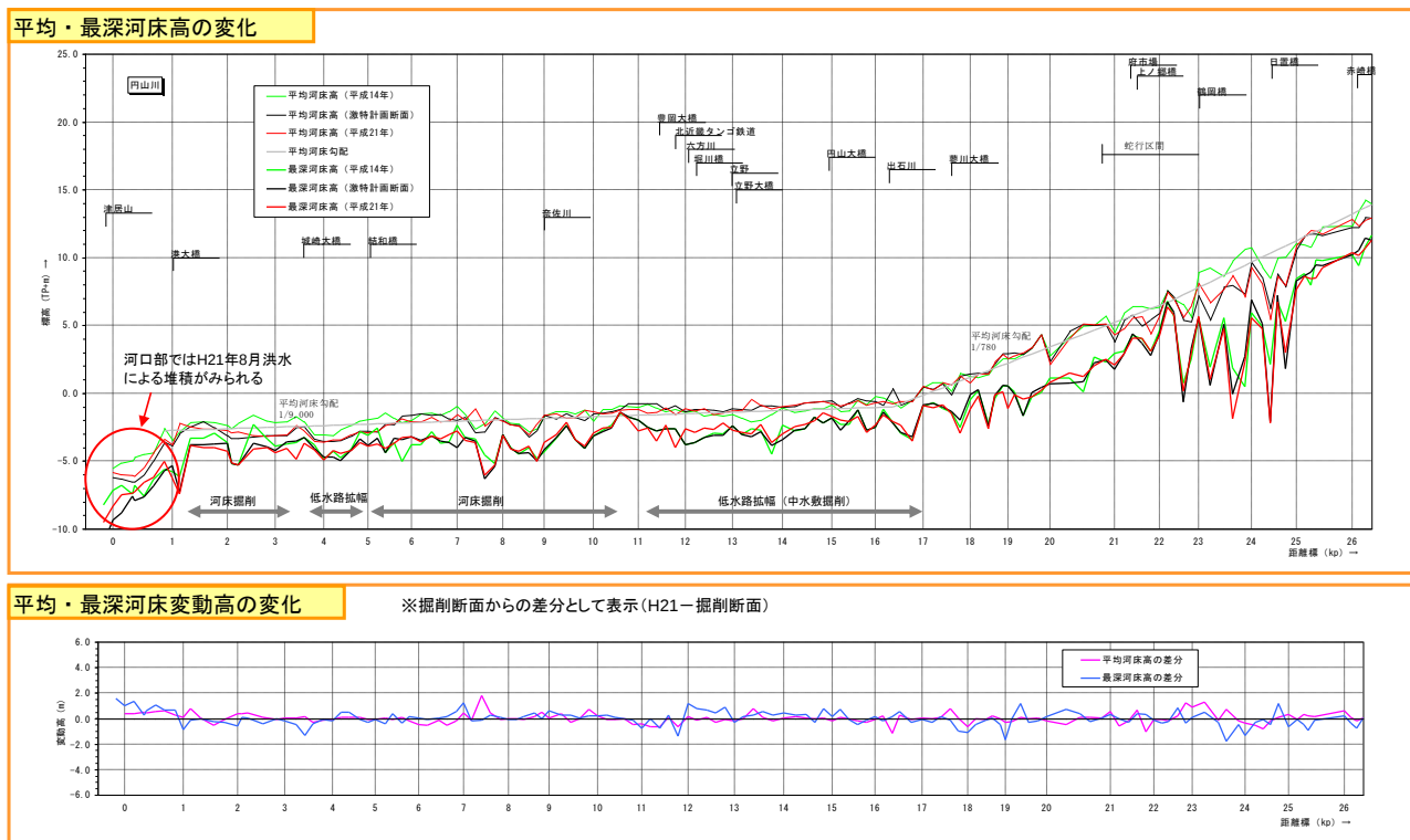
図 1.7 円山川平均河床高縦断面図
