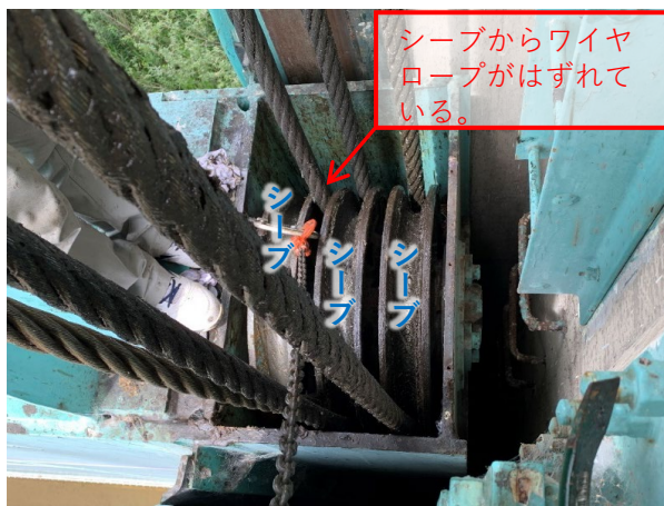
ワイヤロープがシーブからずれた状況（令和6年6月）
