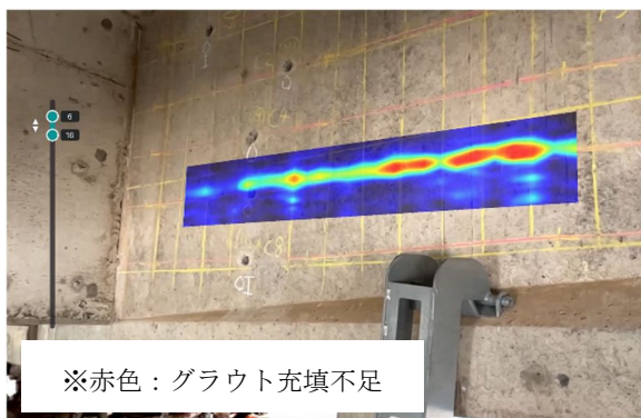
超音波探傷結果 3D 表示例 (AR 表示)
