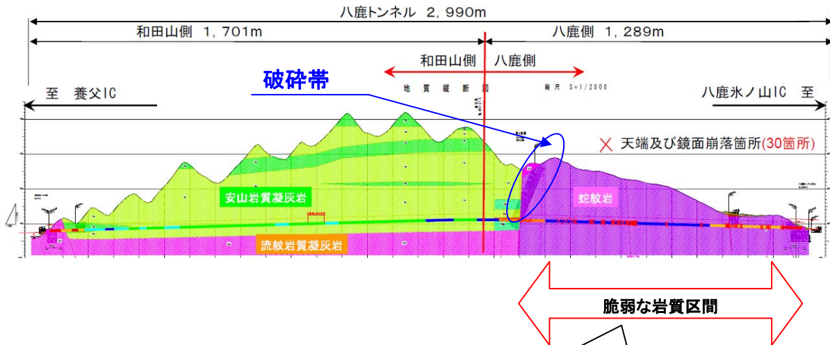
【八鹿トンネルの崩落箇所詳細図】
