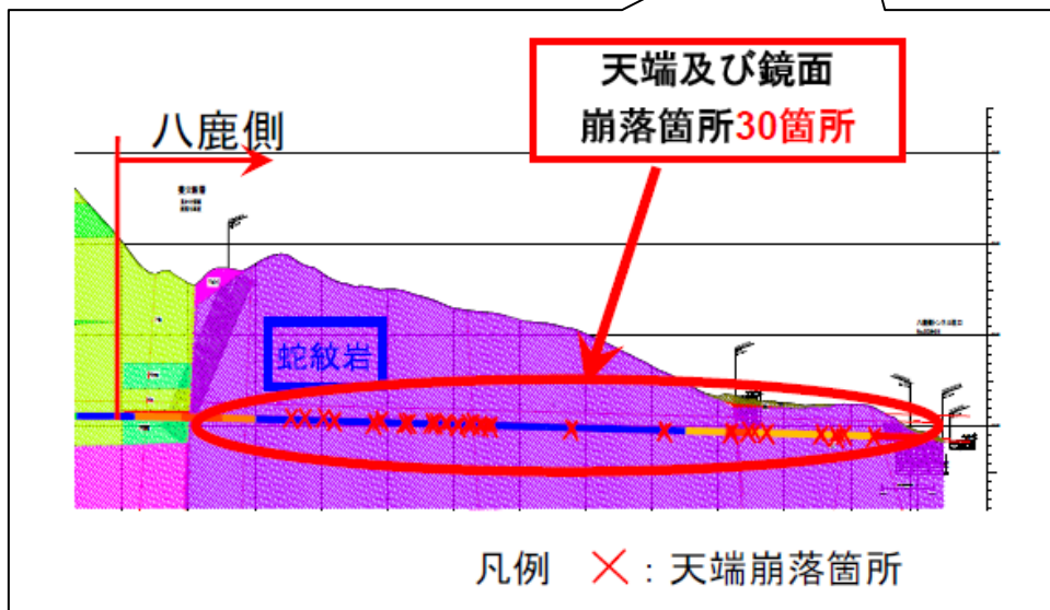
【八鹿トンネルの崩落箇所詳細図】
