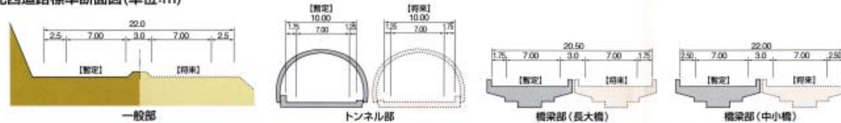
紀北西道路標準断面図(単位:m)
