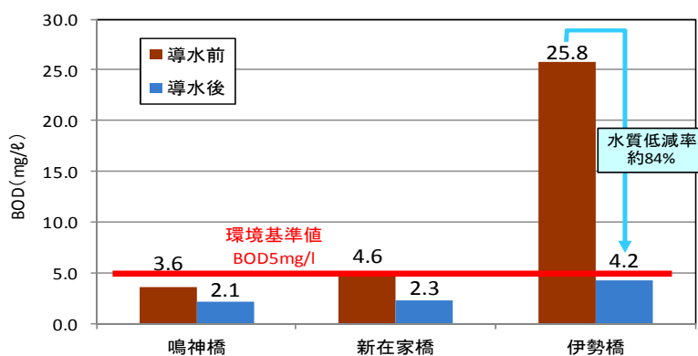
▲大門口川における試験導水前後の水質 (H28)
