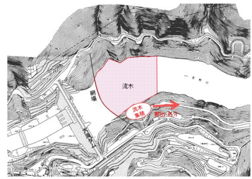
▲大滝ダムにおける流木処理図 (平成30年度の事例)
