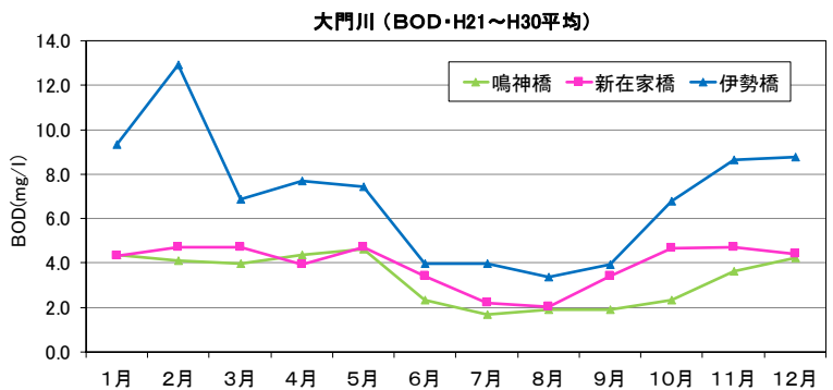
▲大門口川における水質 (月別平均値)
