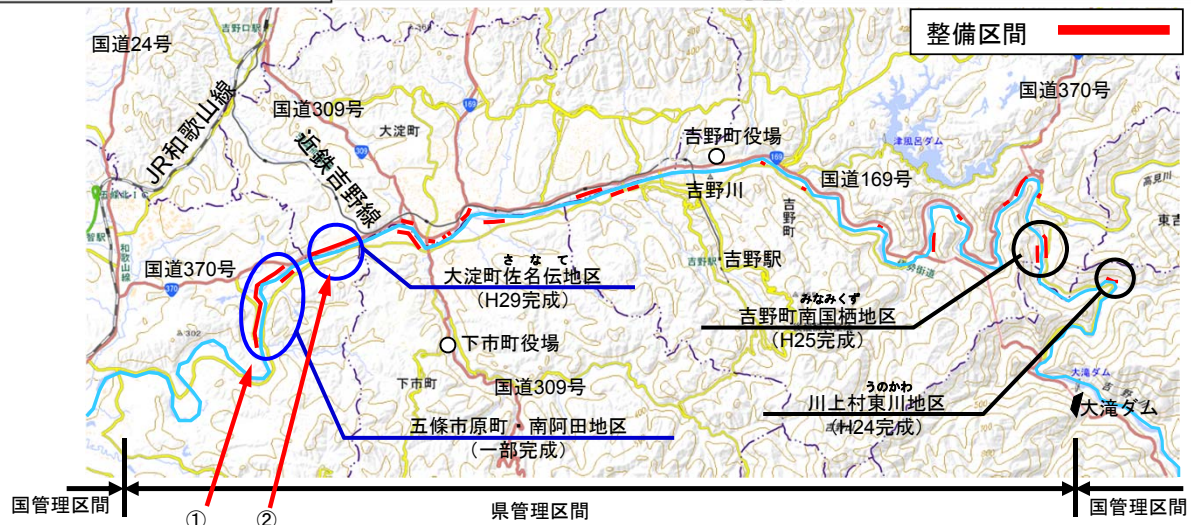
▲整備箇所位置図
