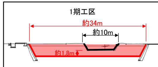
標準断面図
