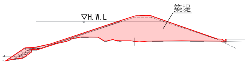
標準断面図(① - ①)
