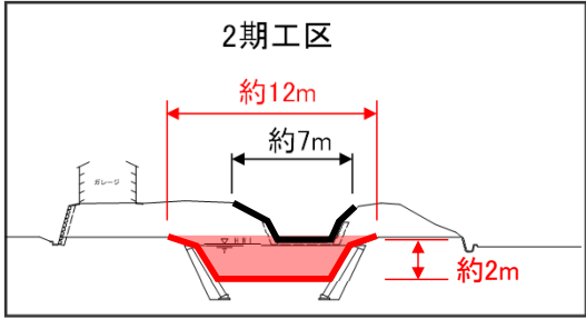
標準断面図
