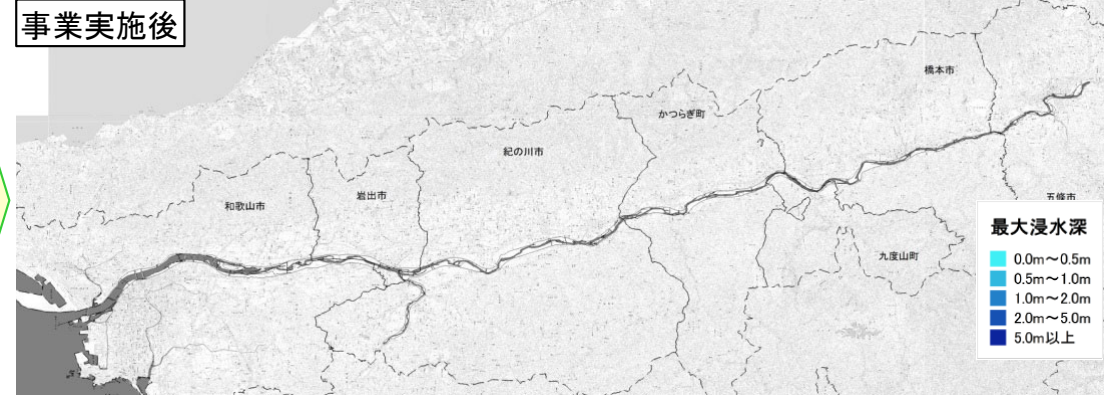
※戦後最大洪水(昭和34年9月洪水)に対する 氾濫解析結果
