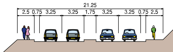
標準断面図[単位:m]
