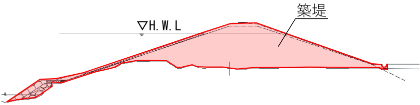
標準断面図(① - ①)
