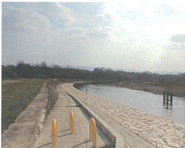
低水護岸の補強
