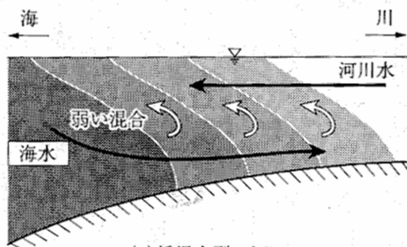
(b) 緩混合型の河口
