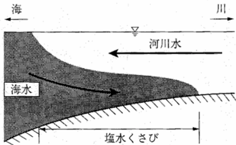
(a) 弱混合型の河口
