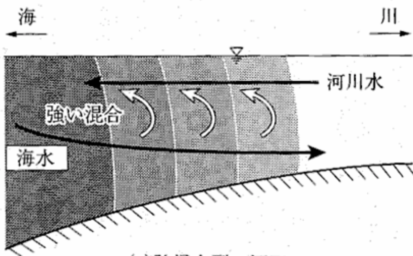
(c) 強混合型の河口
