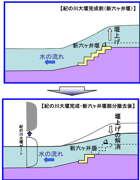
紀の川大堰の完成により洪水時の堰上げが解消され、洪水を安全に流下させることが可能となる。
