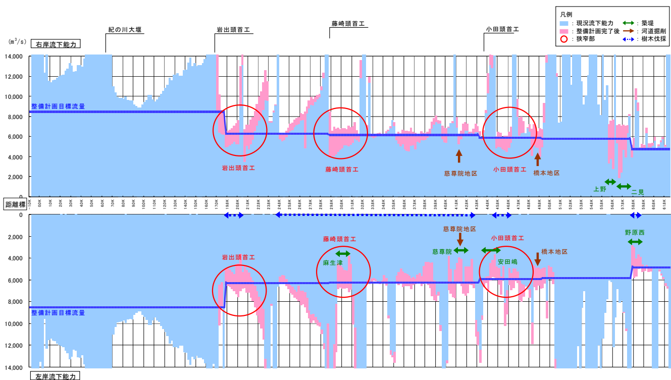
図 4.1.2 整備計画完了時の流下能力
