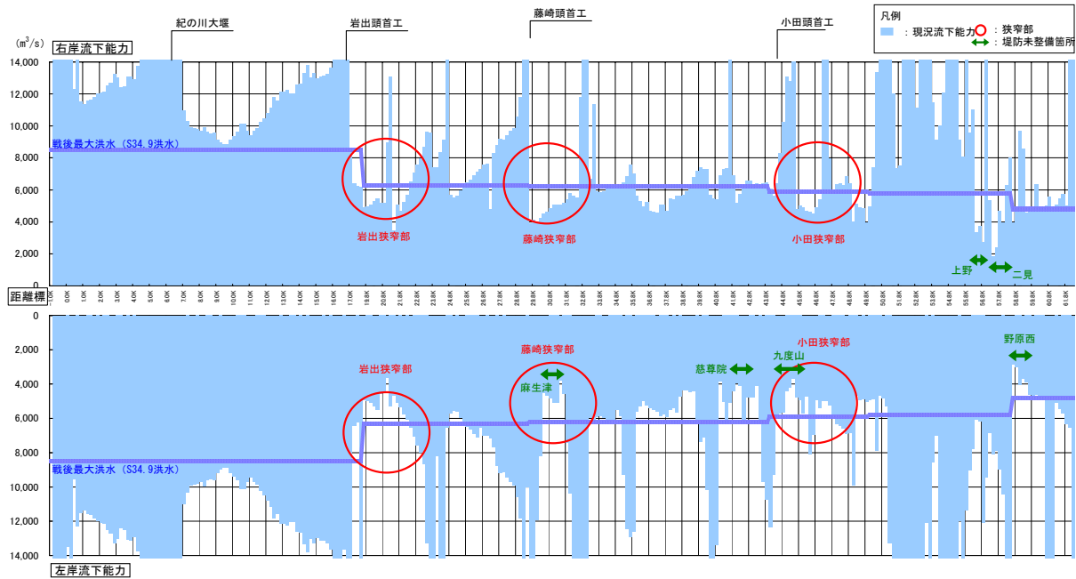
図 2.1.1 現況流下能力
