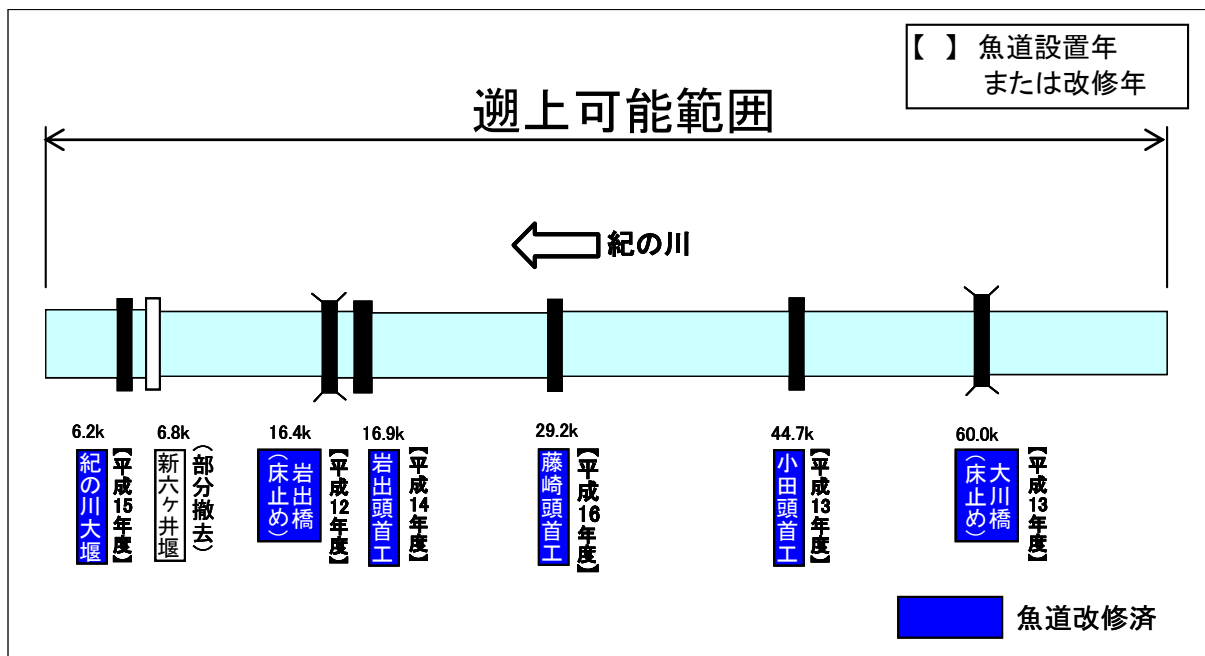
図 2.3.1 魚道の現状
