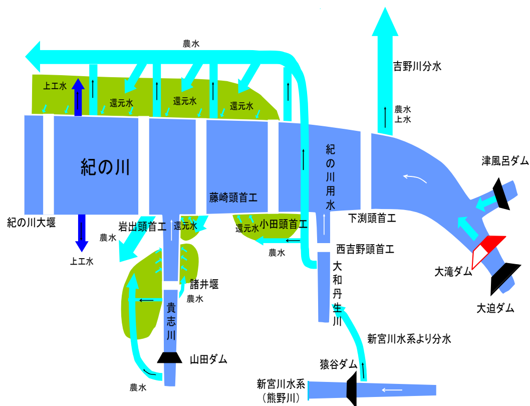
図 1.2.2 利水概要図
