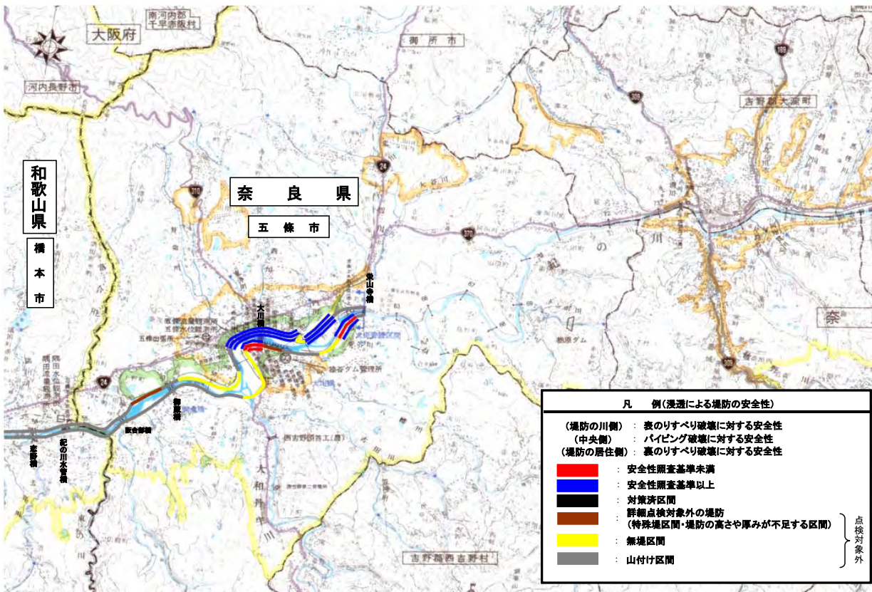
図 2.1.5 紀の川堤防詳細点検結果情報図(平成 23 年 3 月) (4 / 4)
