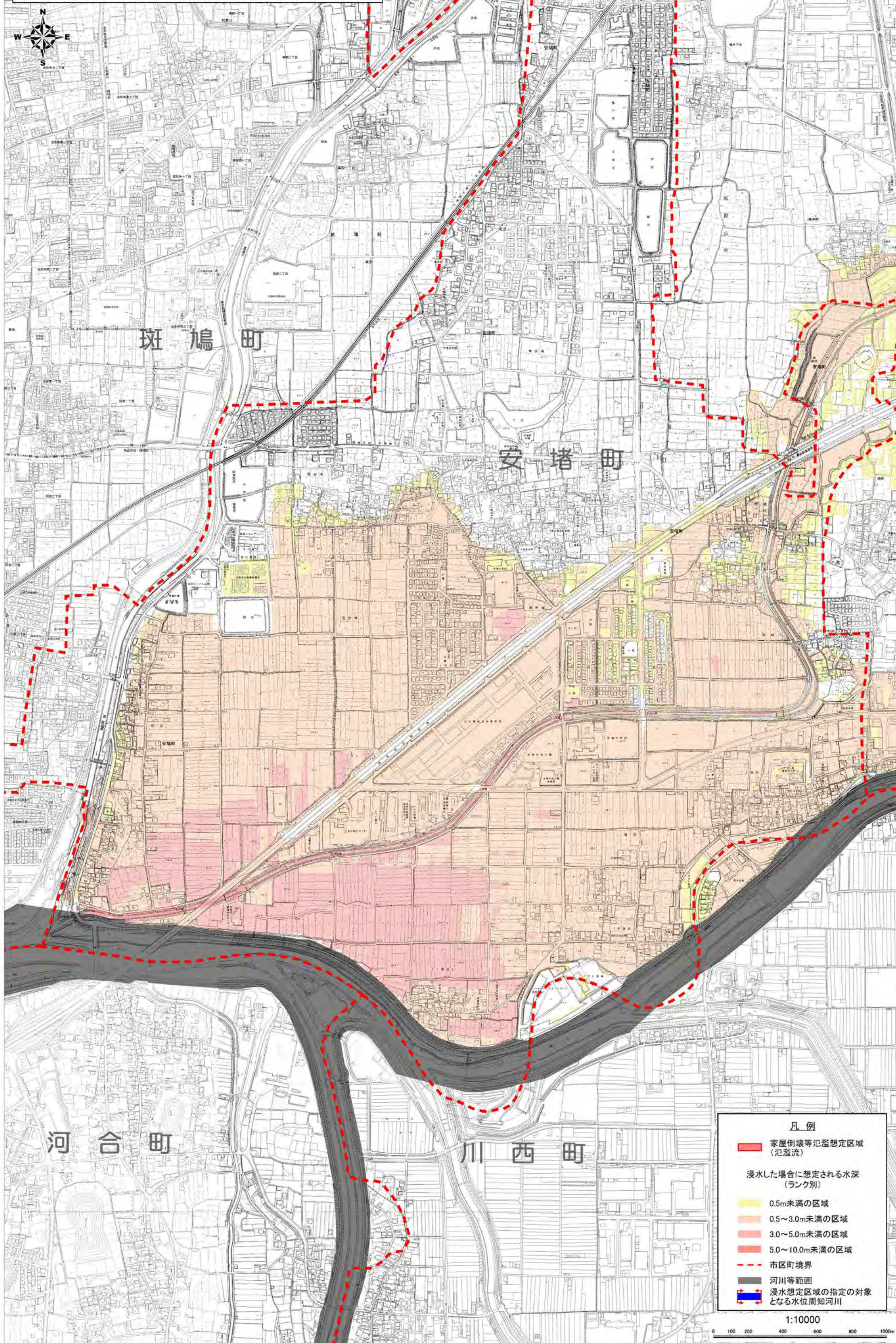
大和川水系佐保川洪水浸水想定区域図(3) (家屋倒壊等氾濫想定区域(氾濫流))
