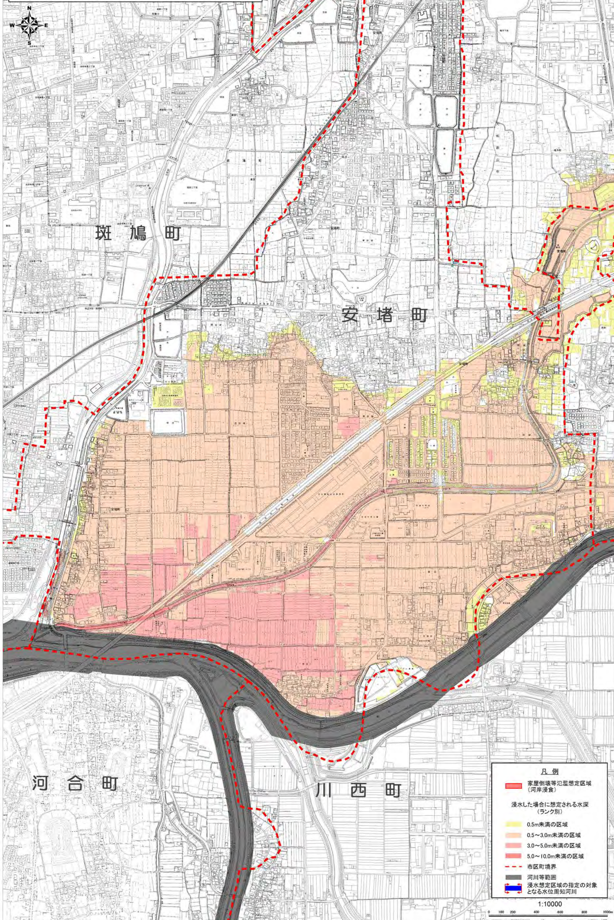
大和川水系佐保川洪水浸水想定区域図(3) (家屋倒壊等氾濫想定区域(河岸浸食))
