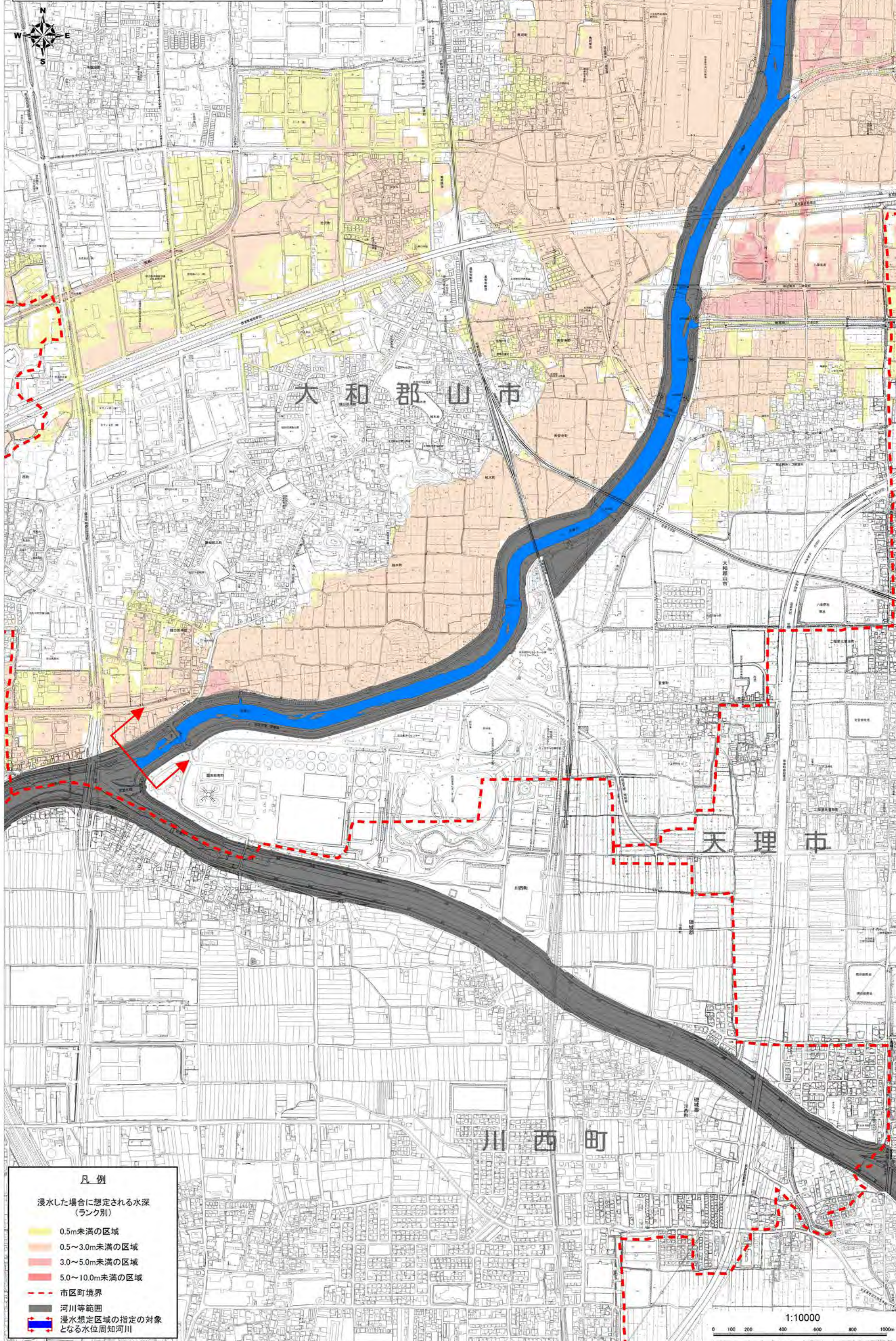
大和川水系佐保川洪水浸水想定区域図(4) (計画規模)
