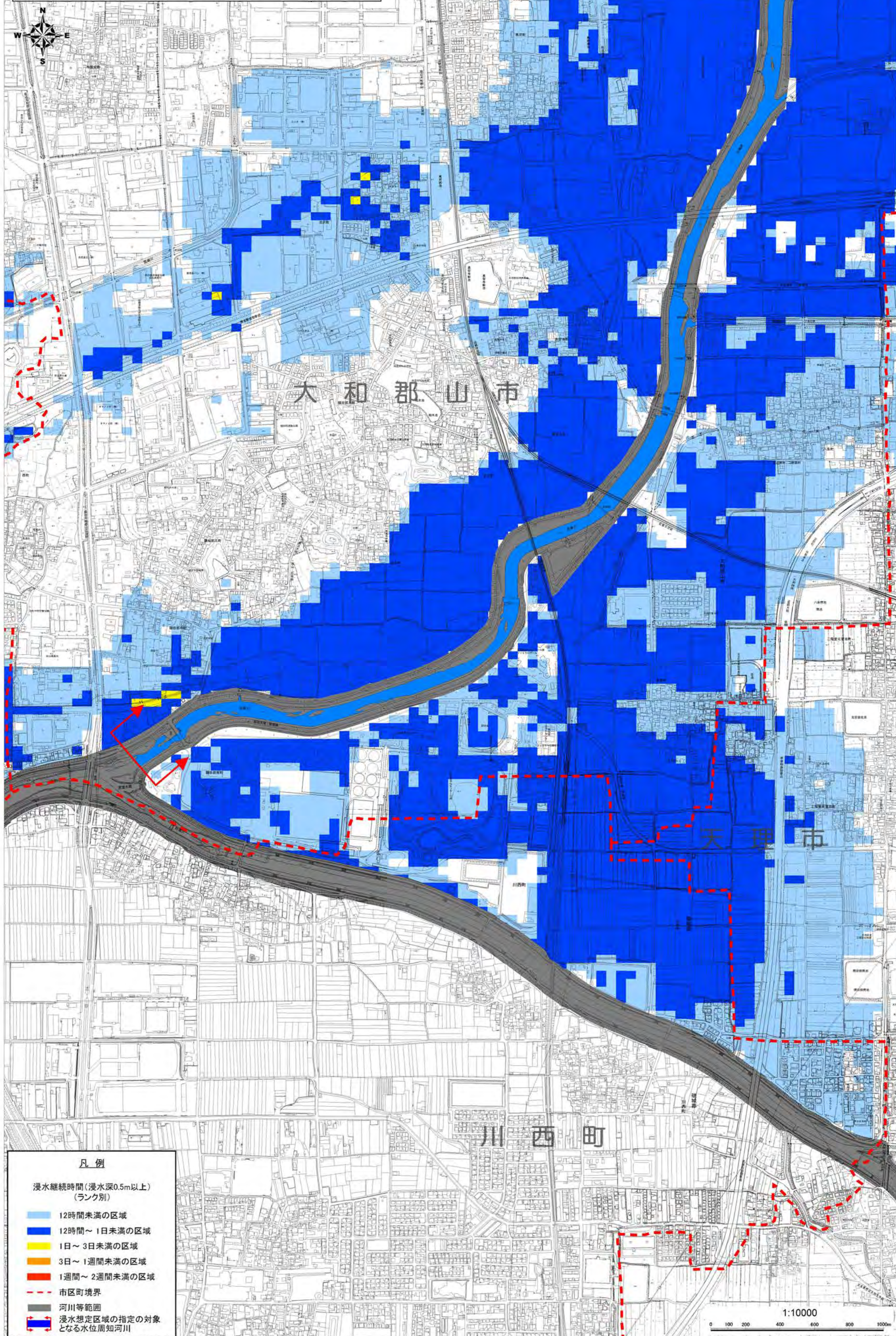
大和川水系佐保川洪水浸水想定区域図(4) (浸水継続時間)
