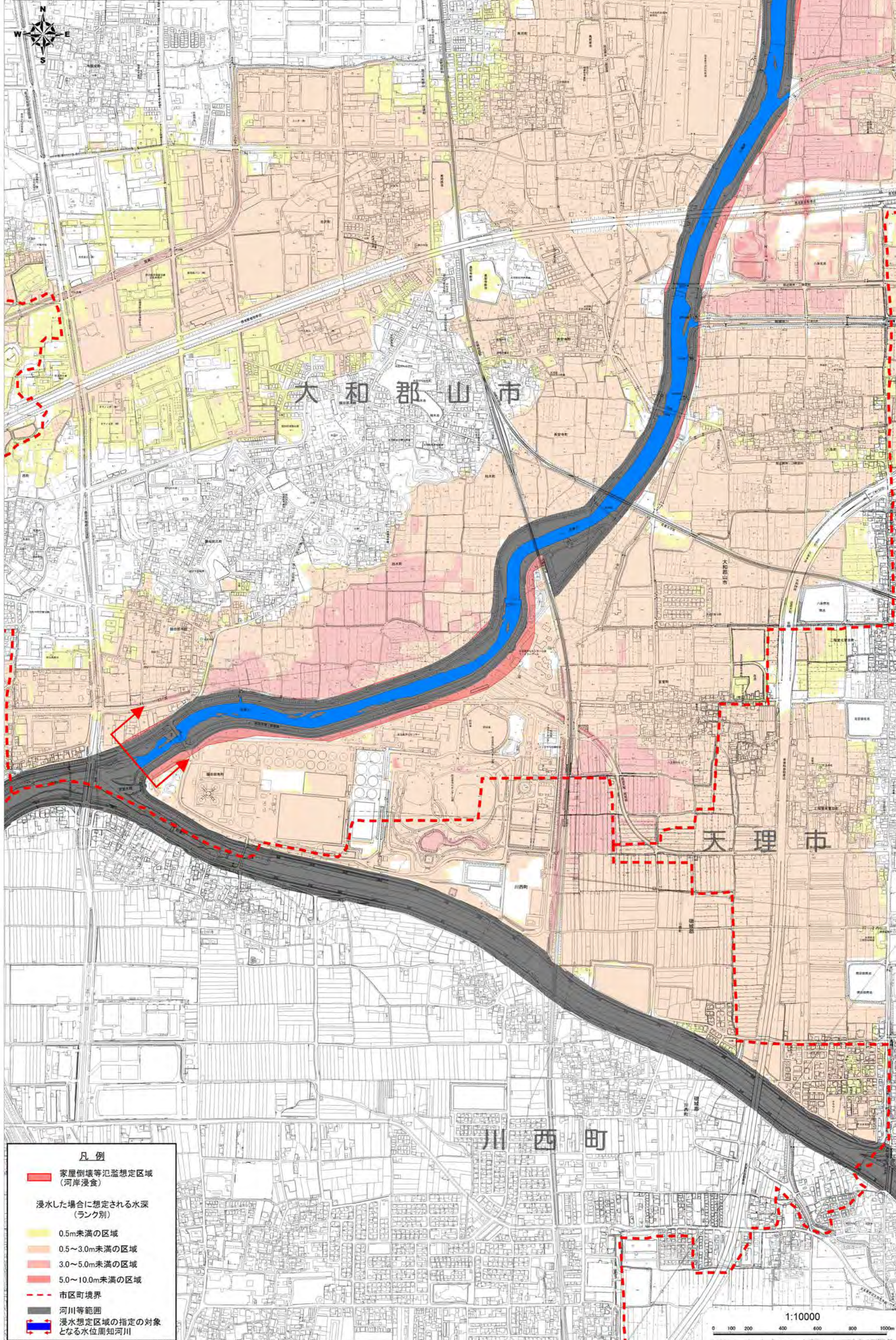
大和川水系佐保川洪水浸水想定区域図(4) (家屋倒壊等氾濫想定区域(河岸浸食))
