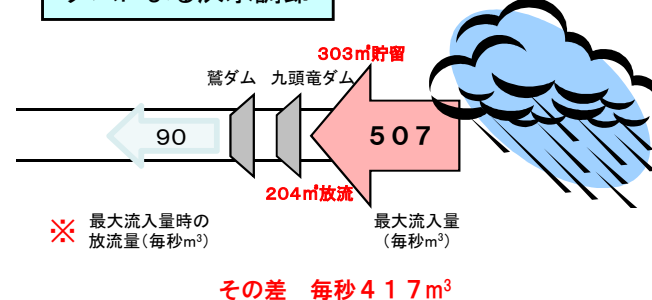
ダムによる洪水調節
