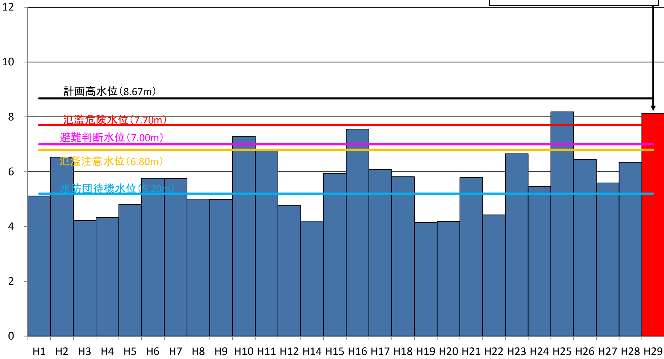
■ 既往洪水での北川(高塚水位観測所)における水位 水位(m)
