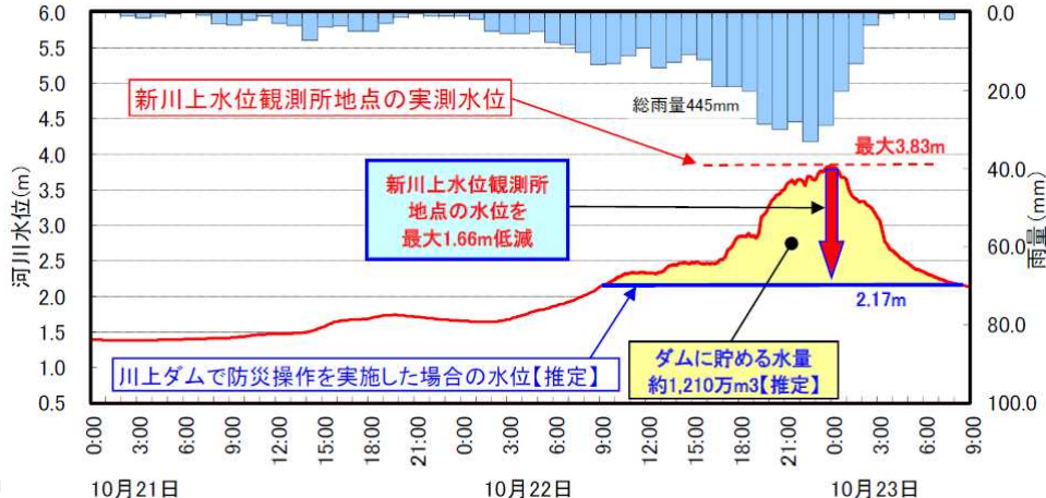
川上ダム流域の降雨量と川上ダム防災操作図(推定) ※新川上位観測所を川上ダム地点として算定(推定)
