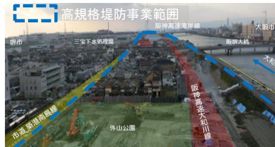
阪神高速大和川線、堺市まちづくり事業と一体整備を行う高規格堤防整備事業地
