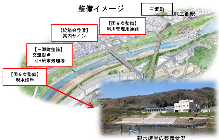
親水護岸の整備状況
