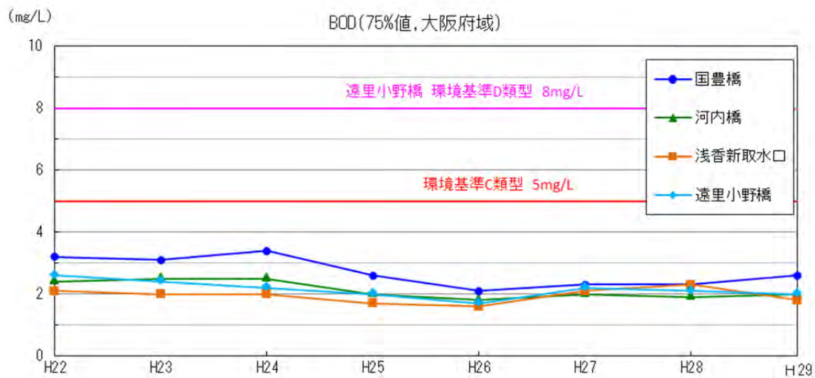
図 4.1.2 本川（大阪府域）地点別 年度 BOD75%値の推移 (H22～H29)
