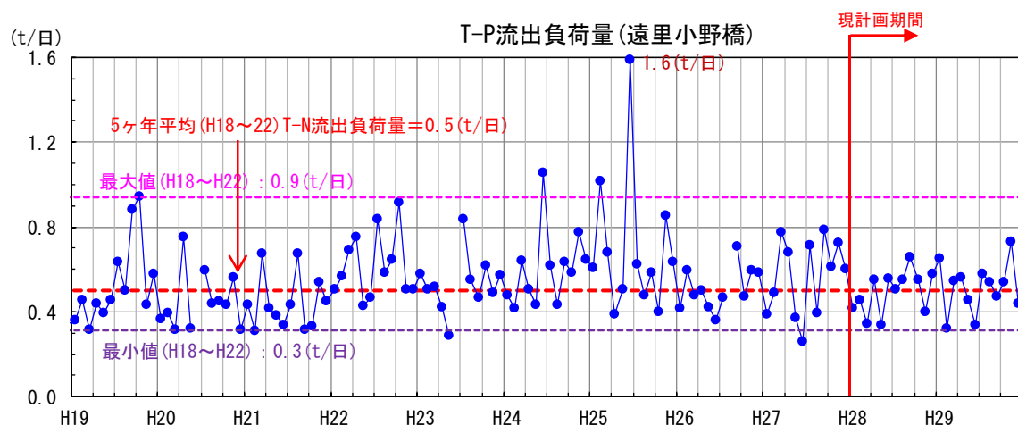
図 5.3.1 大和川本川の T-N 流出負荷量(定期水質調査時)の推移
