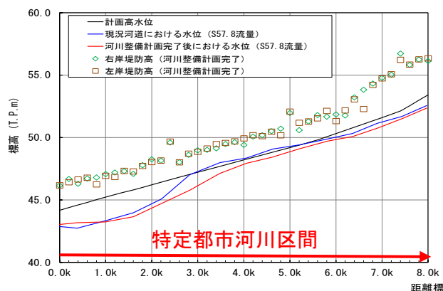
図 4-2 佐保川 水位縦断図
