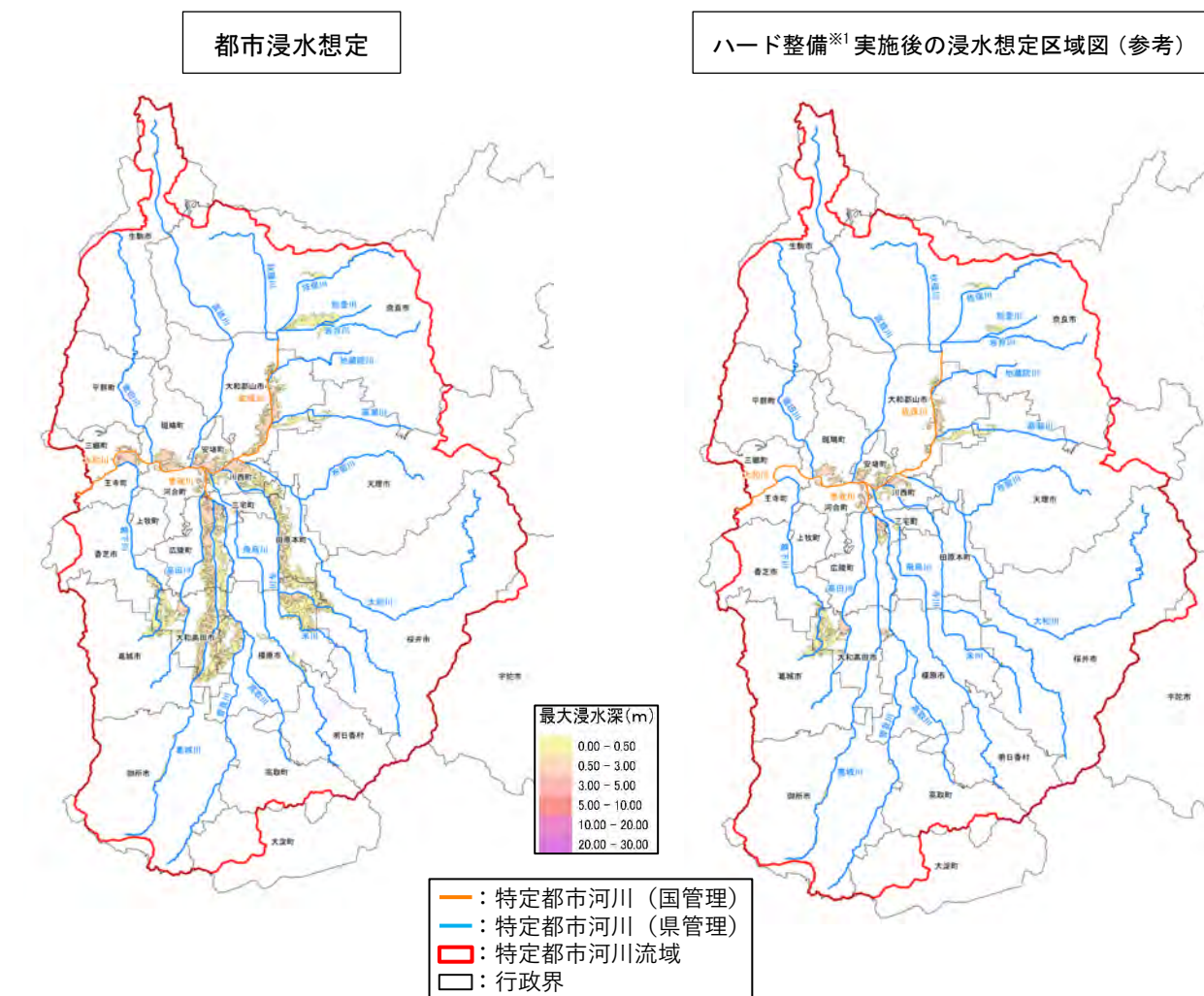
図 3-1 都市浸水想定及びハード整備 ※1 実施後の浸水想定区域図
