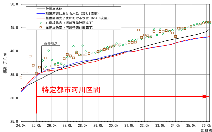
図 4-1 大和川（奈良県） 水位縦断図
