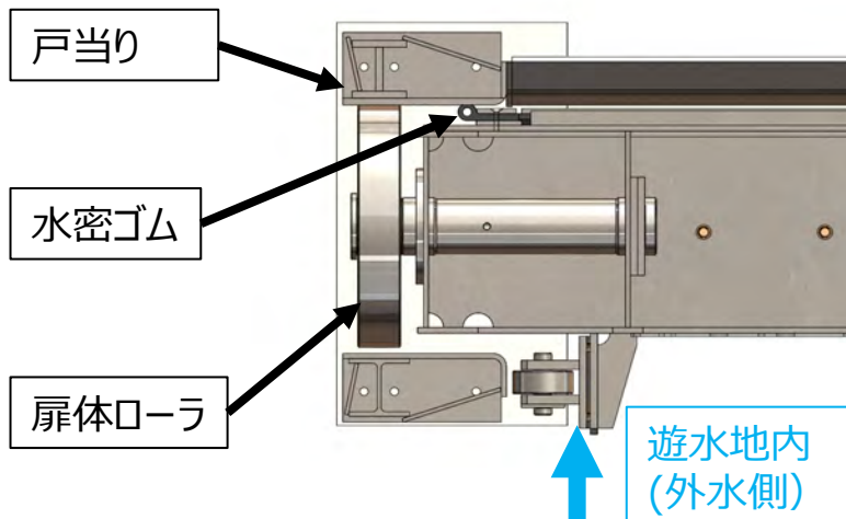
暗渠(内水側)
