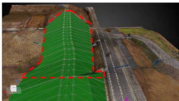
築堤盛土完成予想図
