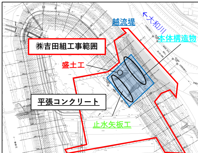
施工平面図
