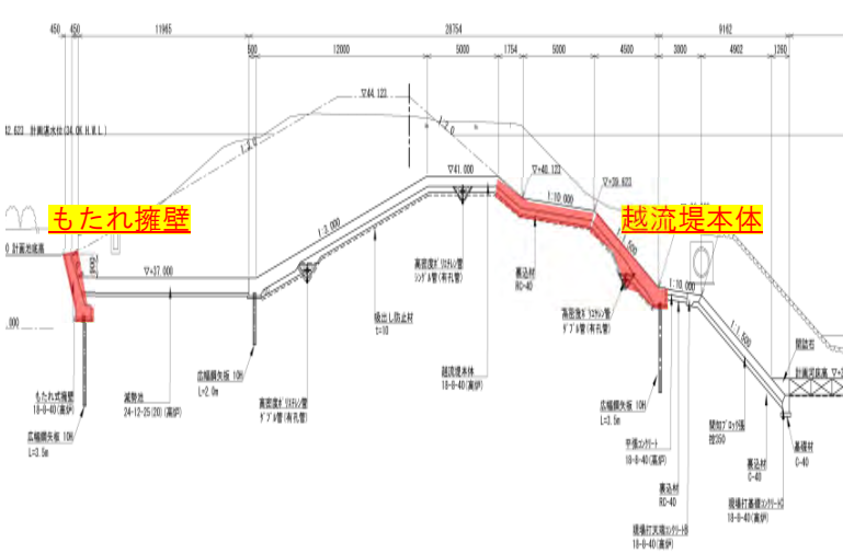
施工断面図
