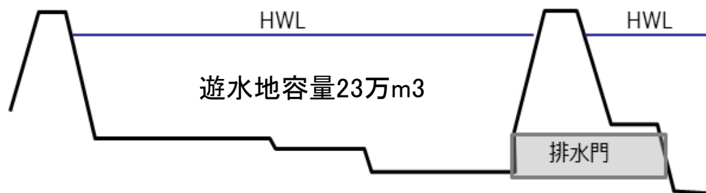
【遊水地の断面イメージ図】
