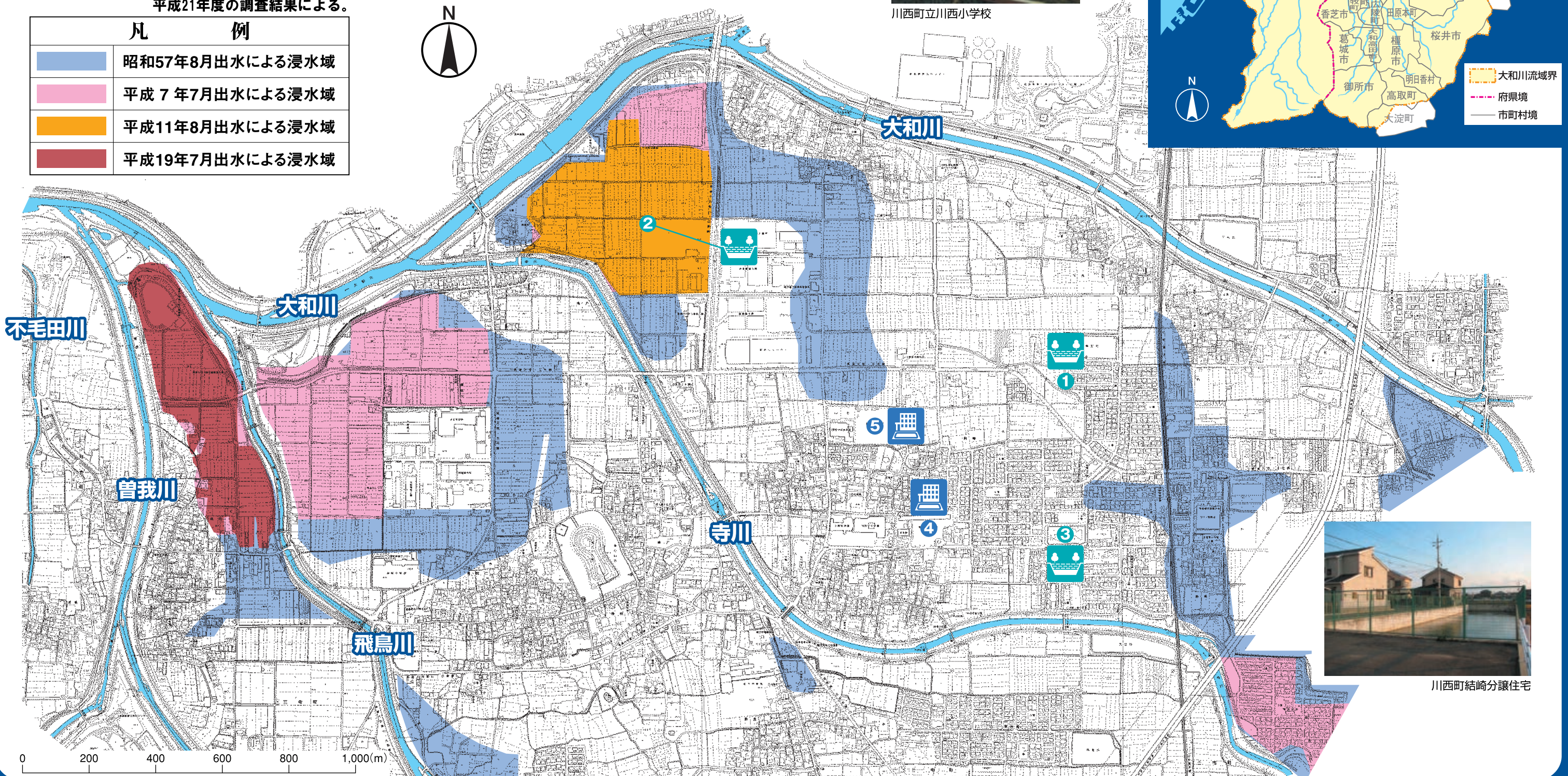
防災調整池
