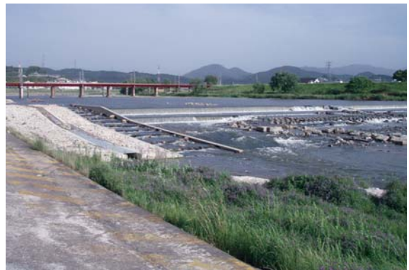
2010 年に完成した柏原堰堤 えんてい の魚道 近鉄道明寺線鉄橋の下流側
