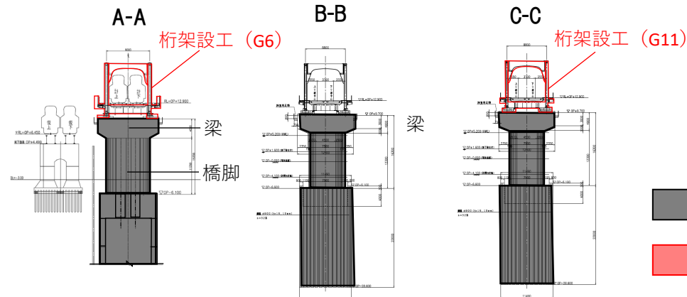
本線断面
