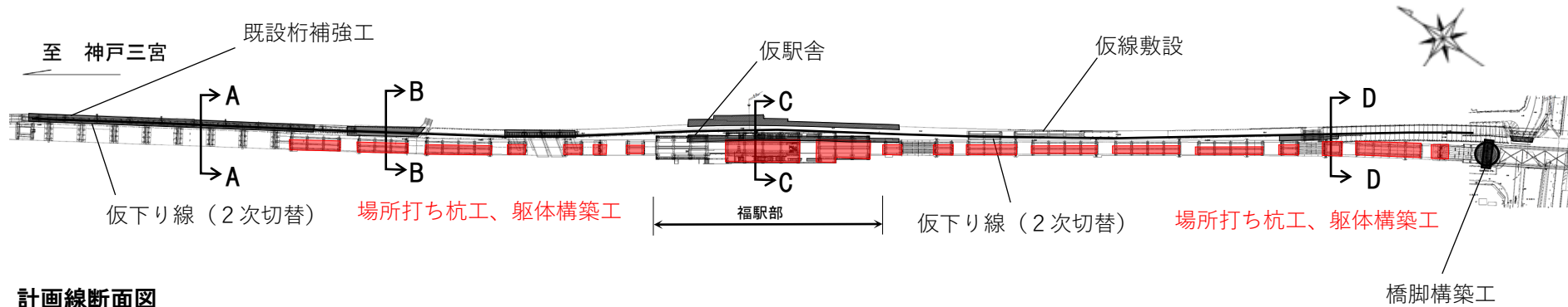
計画線断面図
