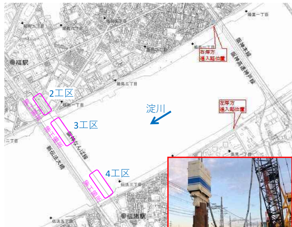
③鋼管矢板井筒基礎工
