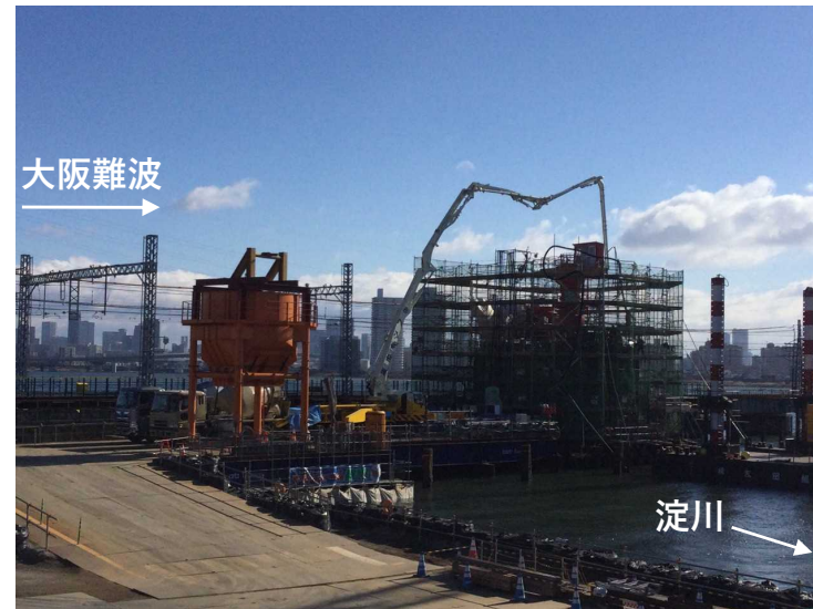
②ニューマチックケーソン基礎工（側壁構築）
