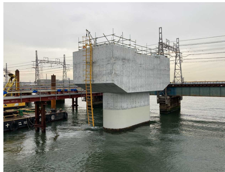
④ P58場所打杭基礎工（フーチング基礎構築）
