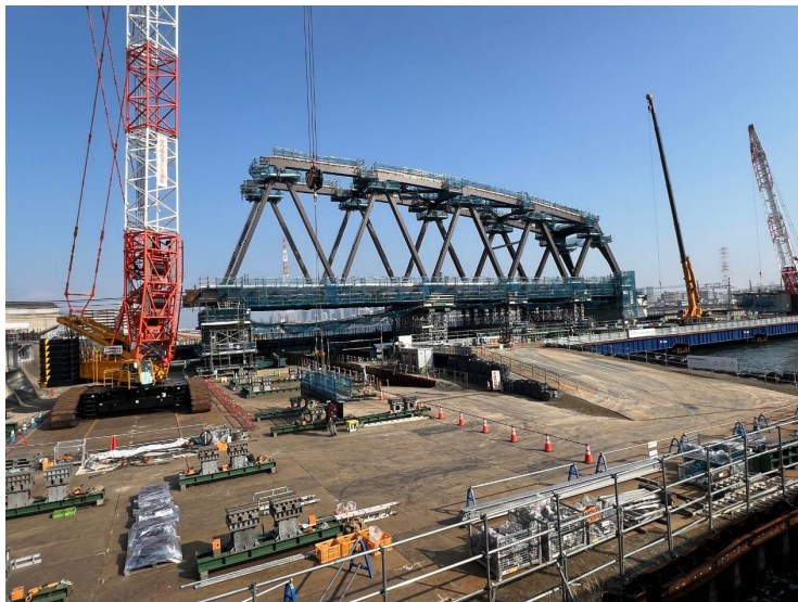
③ 上部工架設工
