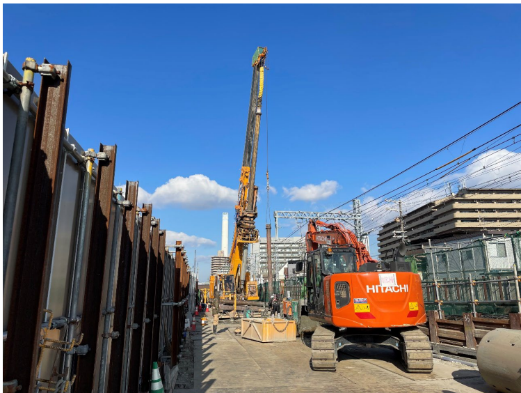
③場所打ち杭工
