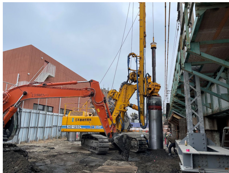
④ボックスカルバート工
