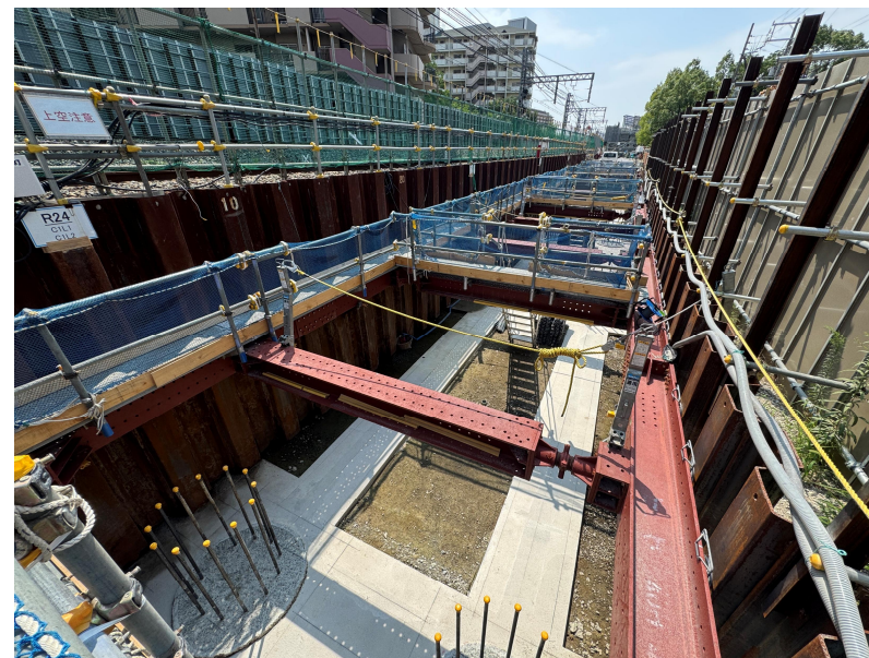
②躯体構築工（地中梁）
