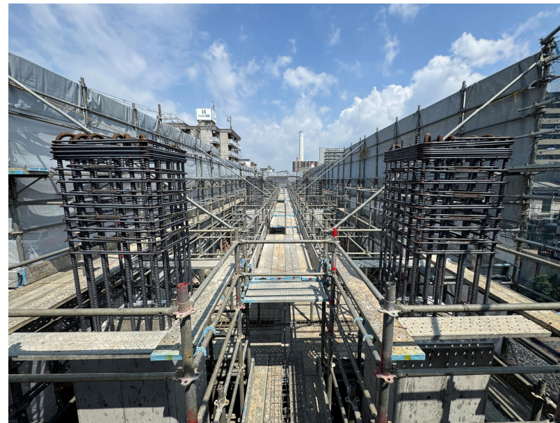
②躯体構築工（柱）
