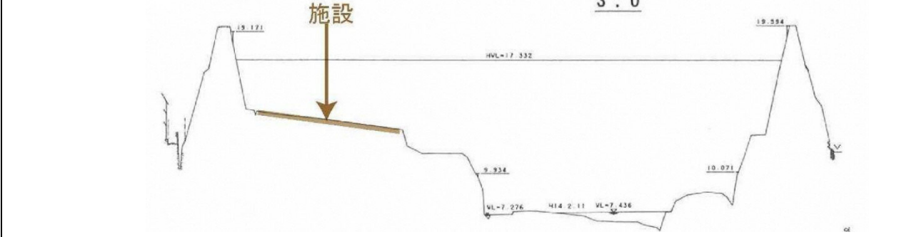
(断面図：3.0k)
